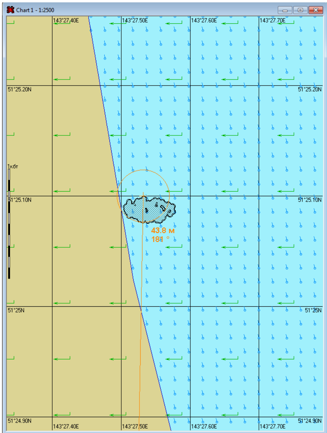
Рис. 2.5. Карта ЧС(Н) на момент достижения нефтяным пятном берега (5ч 15мин) при восточном ветре и скорости ветра 5 м/с.
