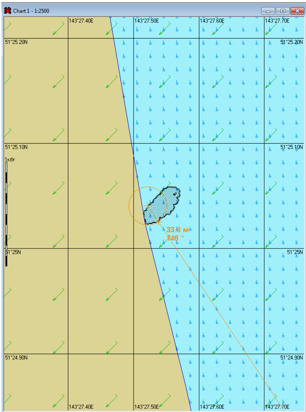
Рис. 2.6. Карта ЧС(Н) на момент достижения нефтяным пятном берега (бч 30мин) при северо-восточном ветре и скорости ветра 5 м/с.
