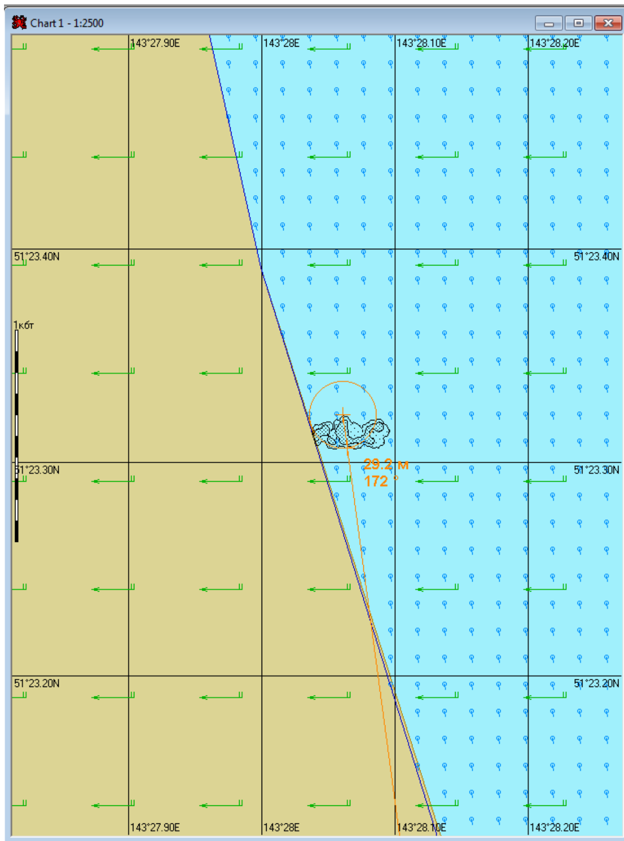
Рис. 2.7. Карта ЧС(Н) на момент достижения нефтяным пятном берега (2ч 35мин) при восточном ветре и скорости ветра 10 м/с.
