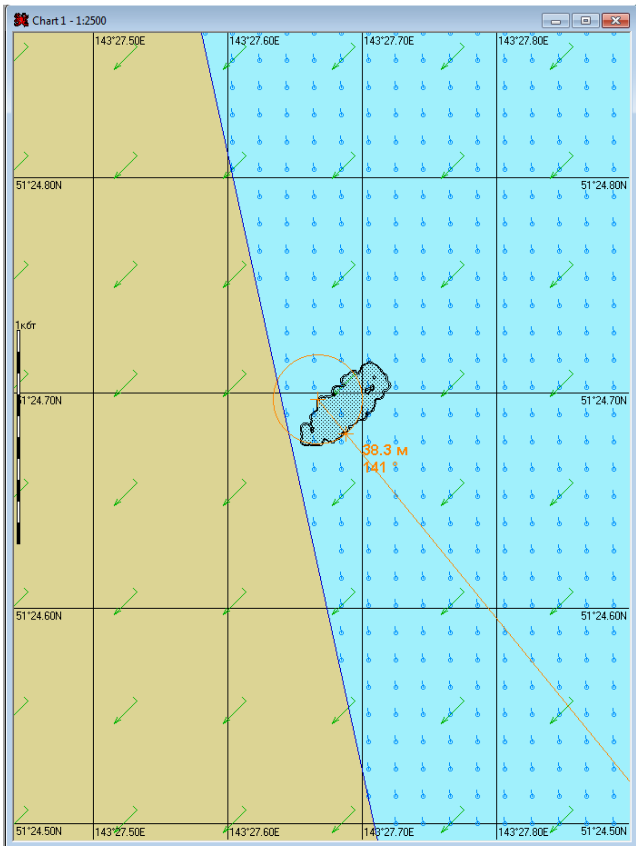
Рис. 2.6. Карта ЧС(Н) на момент достижения нефтяным пятном берега (бч 25мин) при северо-восточном ветре и скорости ветра 5 м/с.
