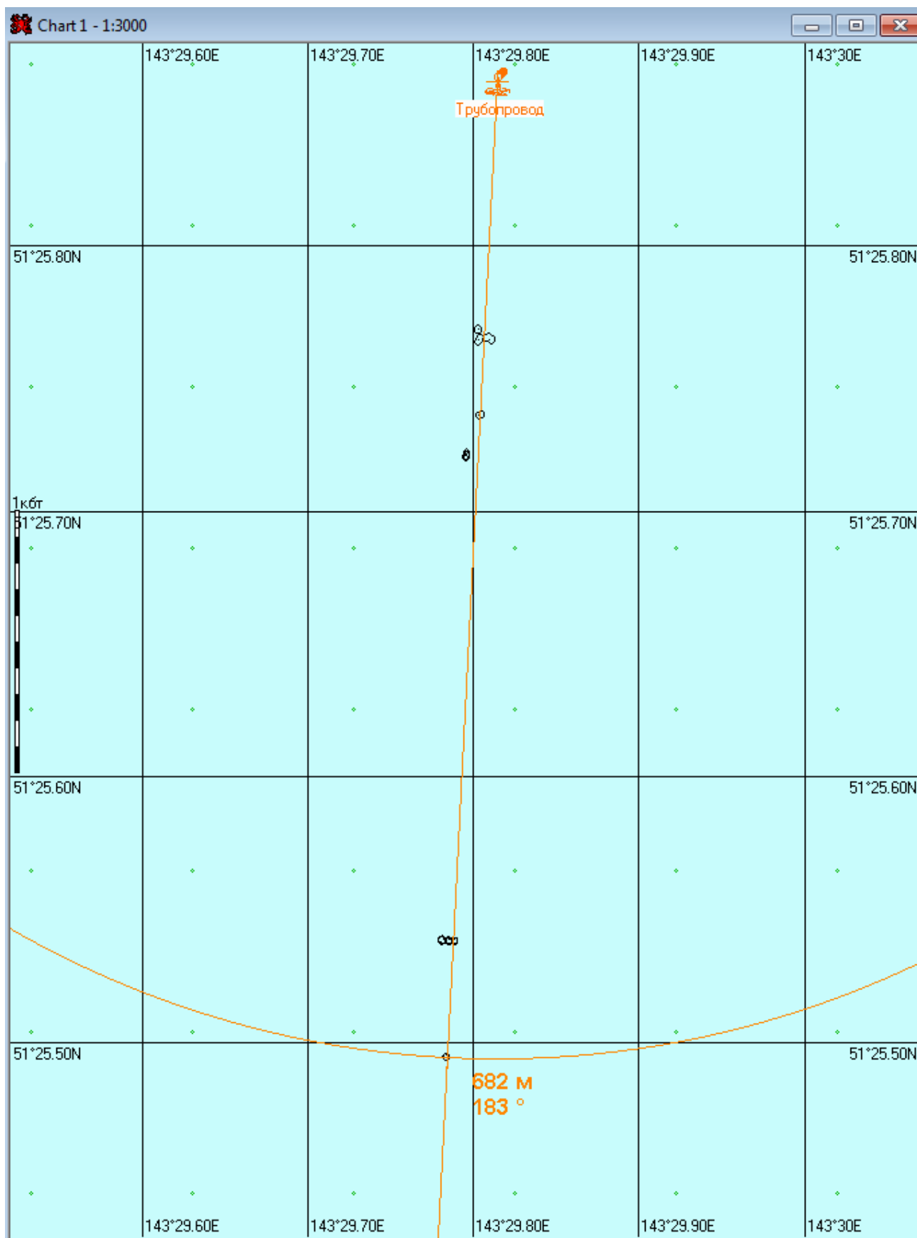
Рис. 1А.3.2. – Карта ЧС(Н) на 3 часа 35 минут с момента разлива (расстояние от источника разлива до дальней кромки) (полное рассеивание)
