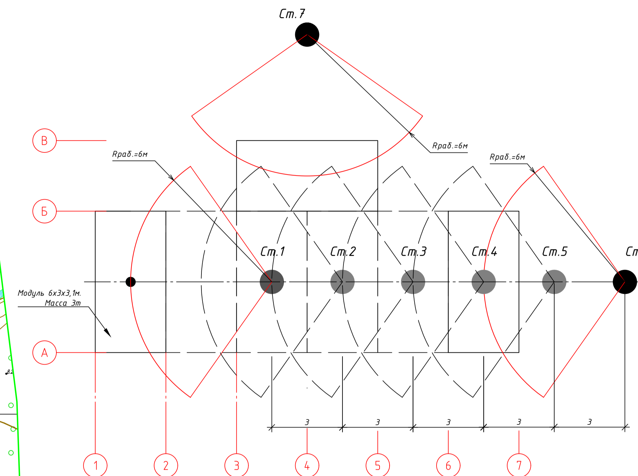
Схема расположения стоянок автокрана
