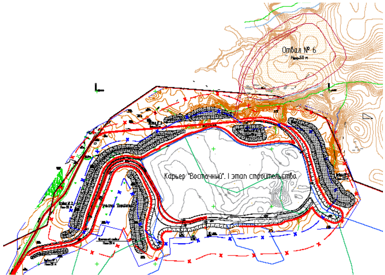
Рисунок 3.1 – Схема размещения вскрышных пород в отвале №6
