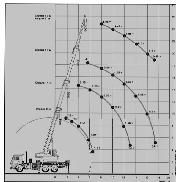
Грузовысотная характеристика крана грузоподъемностью 16т
