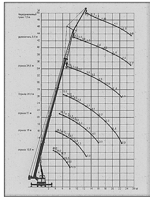
Грузовысотная характеристика крана грузоподъемностью 16т
