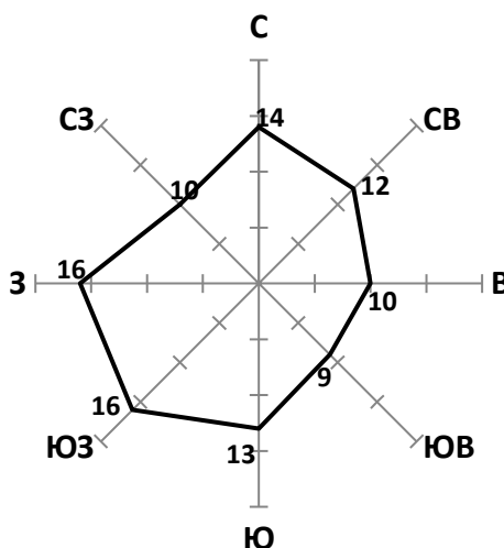
Рисунок 2.2 – Годовая повторяемость направлений ветра, %
