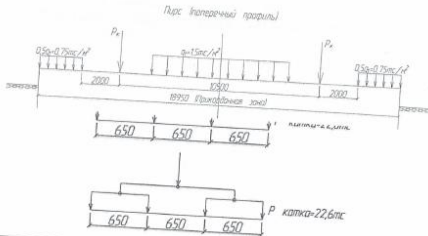
Схема нагрузок
