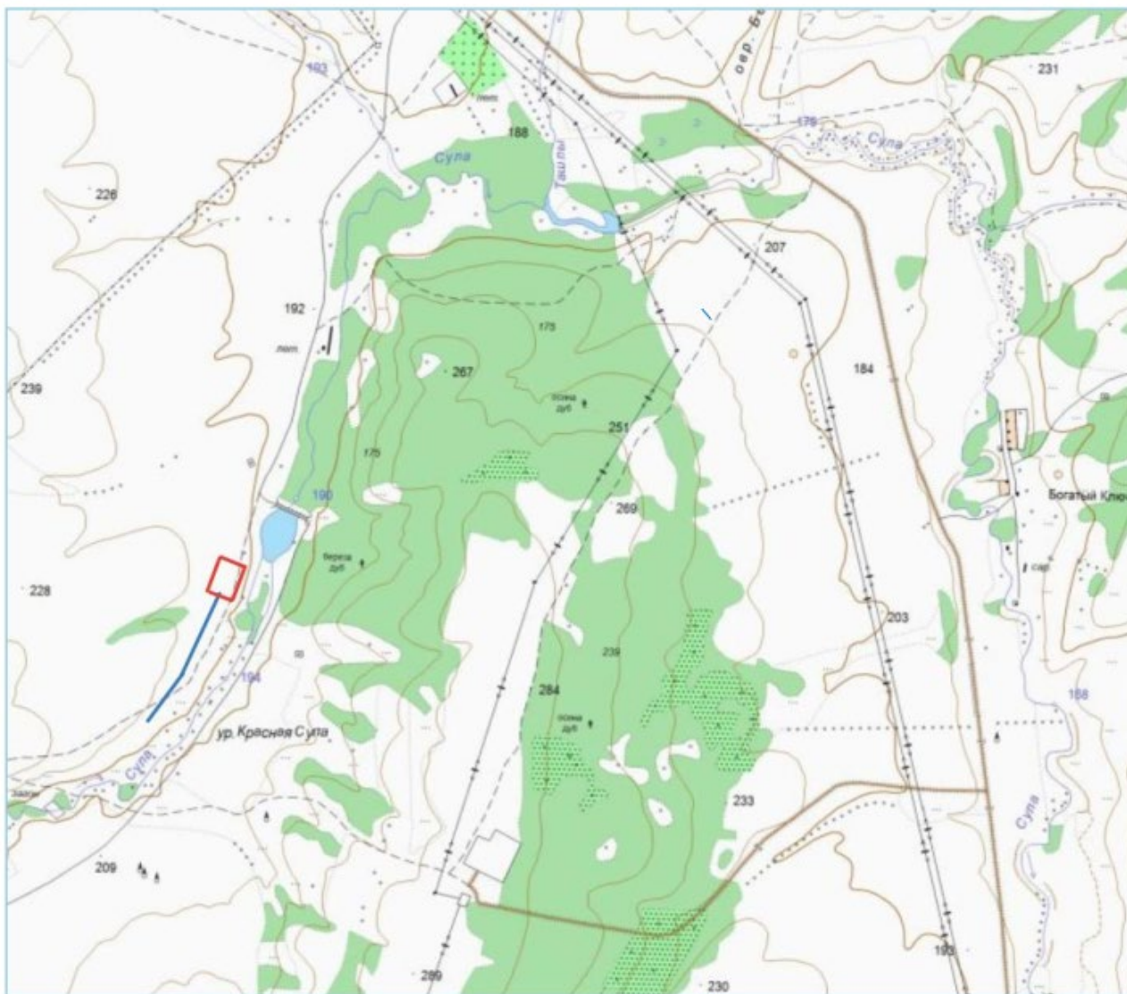
— изыскиваемая трасса нефтегазопровода □ куст скважин №6254
