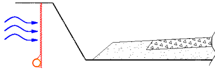
Рис. 16. Перехватывающий дренаж
