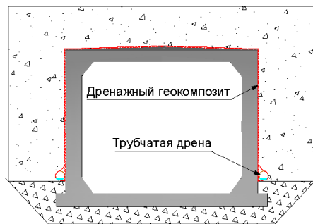
Рис. 19. Дренаж тоннелей
