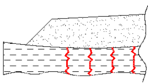
Рис. 20. Применение вертикальных ленточных дрен
