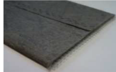
Рис. 11. Рельефная мембрана в виде ленты, скрепленная по контуру геотекстилем
