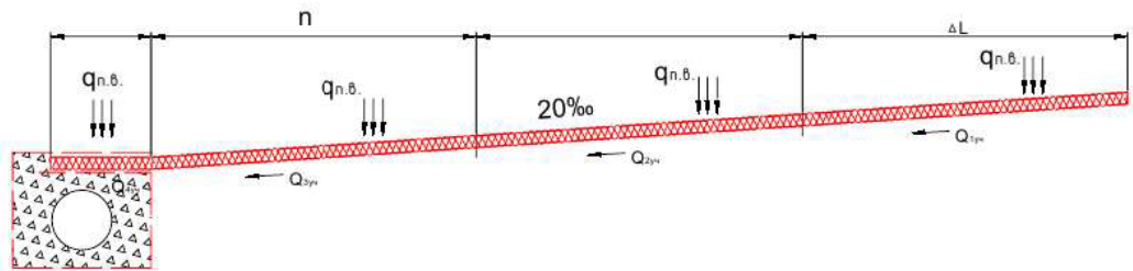
Рис. 26. Схема разбивки дренажной прослойки на участки
