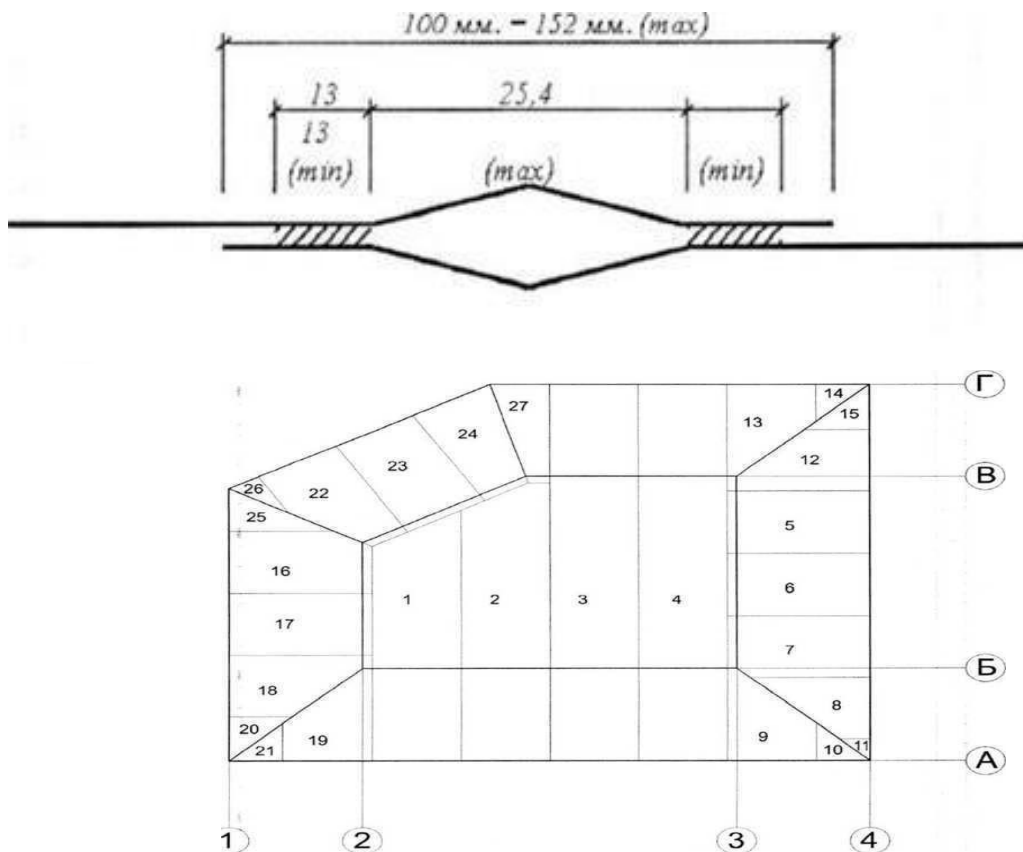
Рис. 2.2 – Технология сварки геомембраны
