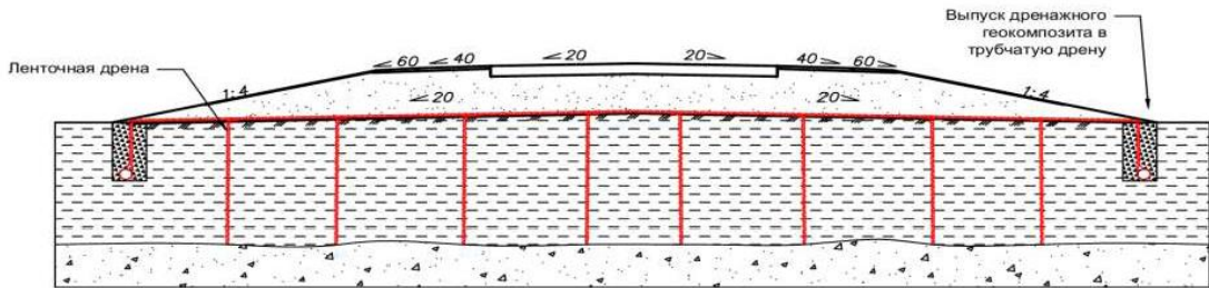
Устройство дренирующей прослойки из дренажного геокомпозита совместно с ленточными дренажами
