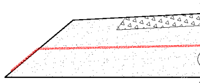
Рис. 15. Горизонтальный пластовый дренаж
