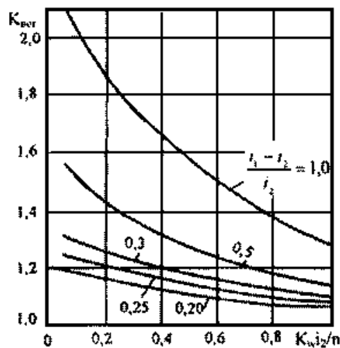
Рис. 25. Номограмма для определения коэффициента K_{вод}
