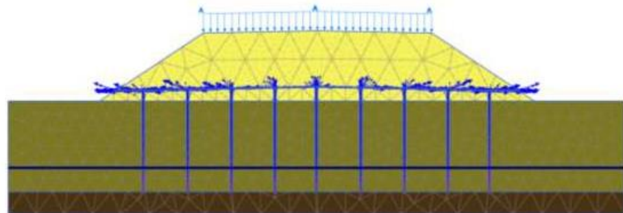
Рис. 34. Направление движения воды в дренажной системе
