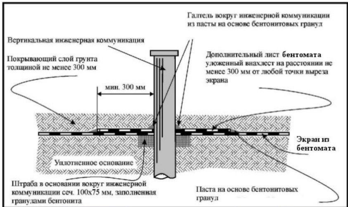
Рис. 4. Осевое сечение вертикальной инженерной коммуникации.
