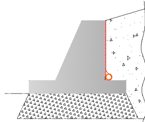
Рис. 17. Дренаж подпорных стен
