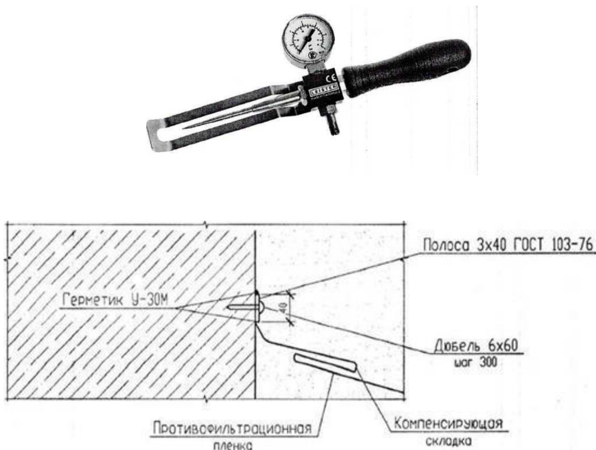
Рис. 2.3 – Примыкания к бетонным конструкциям
