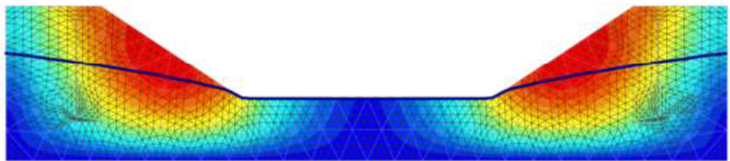
Рис. 30. Потеря устойчивости подтопленного откоса выемки
