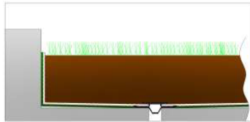
Рис. 21. Дренаж при устройстве зеленых крыш
