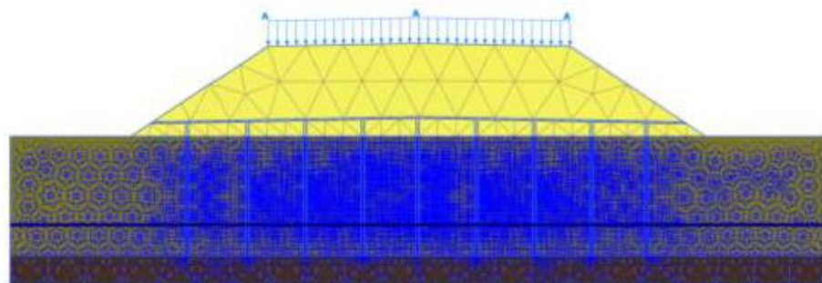
Рис. 32. Распределение избыточного порового давления в слабом основании
