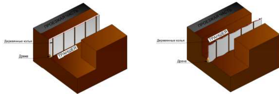
Рис. 40. Монтаж дренажного мата в траншее
