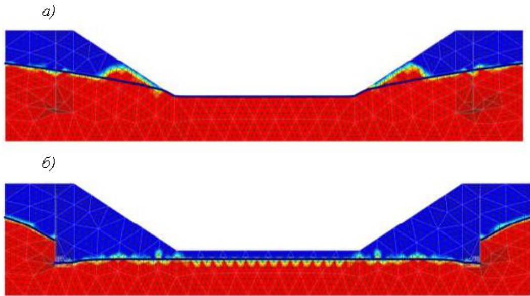
Рис. 31. Исходное (а) и конечное (б) положение уровня грунтовых вод при работе дренажного геокompозита
