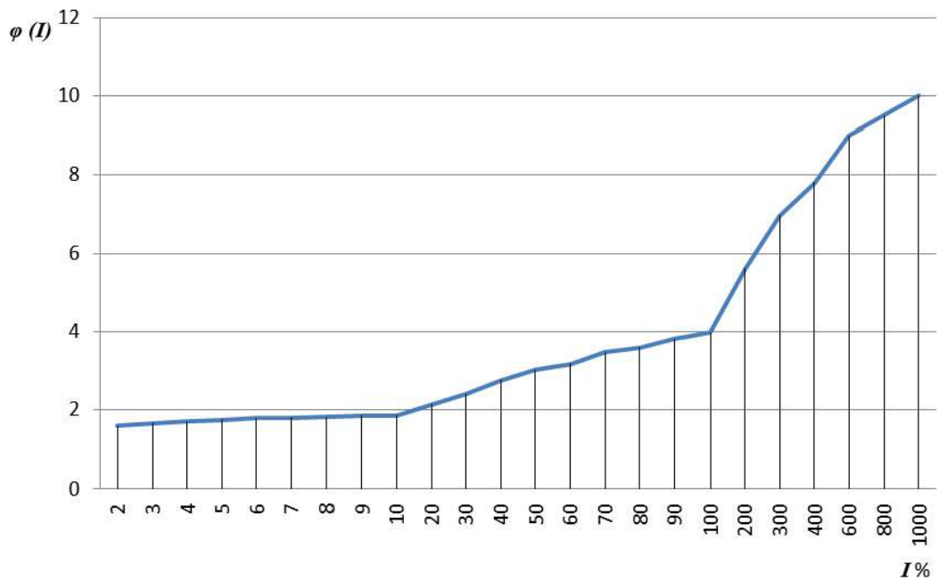
Рис. 24. График определения функции уклона \varphi(I)
