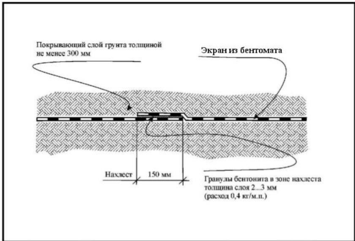
Рис. 3. Герметизация зоны нахлеста.
