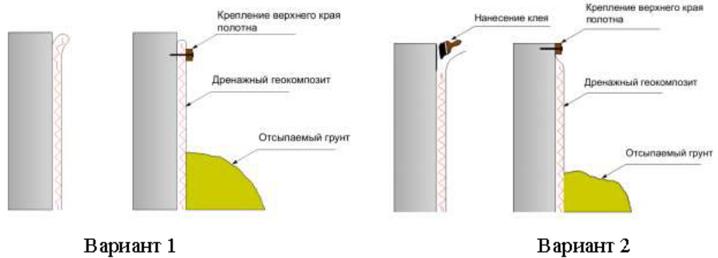
Рис. 43. Крепление дренажного геокомпозита к стене
