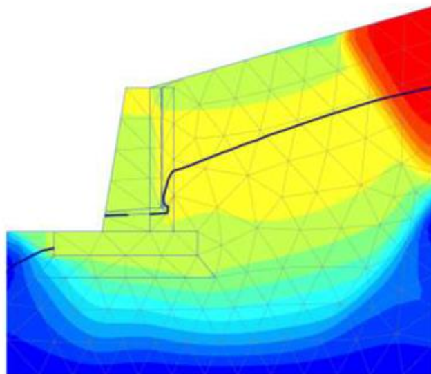
Рис. 36. Распределение перемещений после дренаживания
