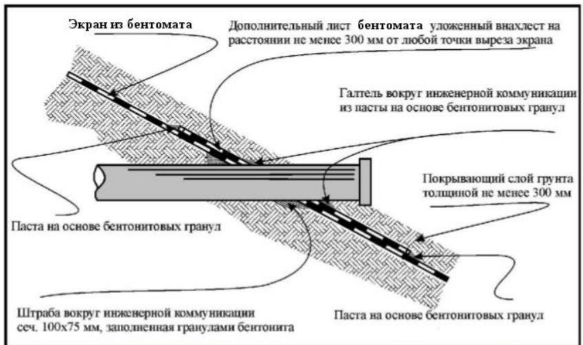
Рис. 5. Осевое сечение горизонтальной инженерной коммуникации.
