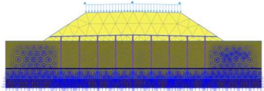
Рис. 33. Распределение избыточного порового давления после устройства дренажа
