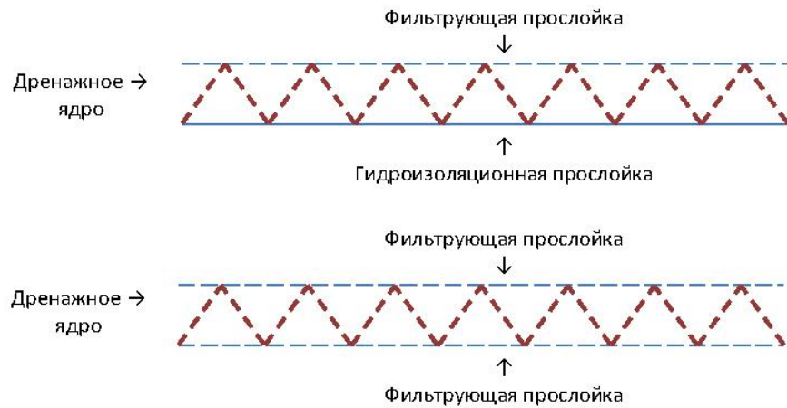
Рис. 1. Виды дренажных геоконпозитов
