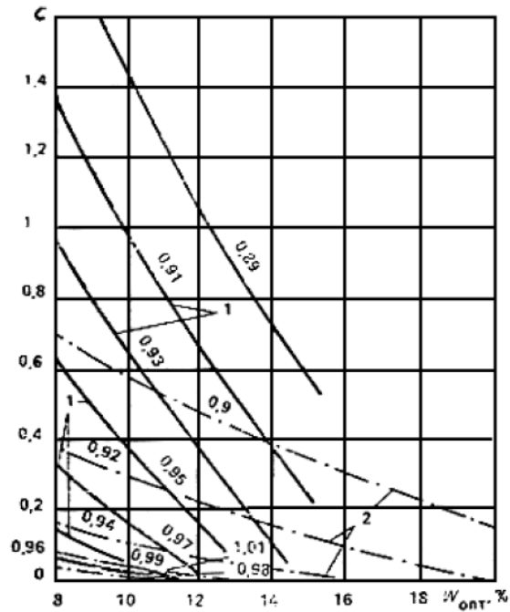
1 - супеси; 2 - суглинки и глины, цифры на кривых - коэффициенты уплотнения грунта
