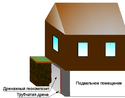
Рис. 18. Вертикальный пристенный дренаж
