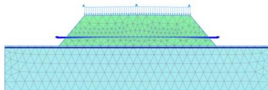
Рис. 29. Направление движения воды с применением прослойки дренажного геокompозита
