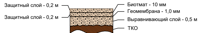
Узел В. Конструкция рекультивационного покрытия
