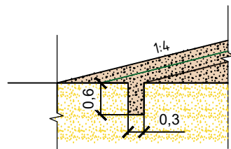
Узел Б. Анкерная траншея крепления биоматов
