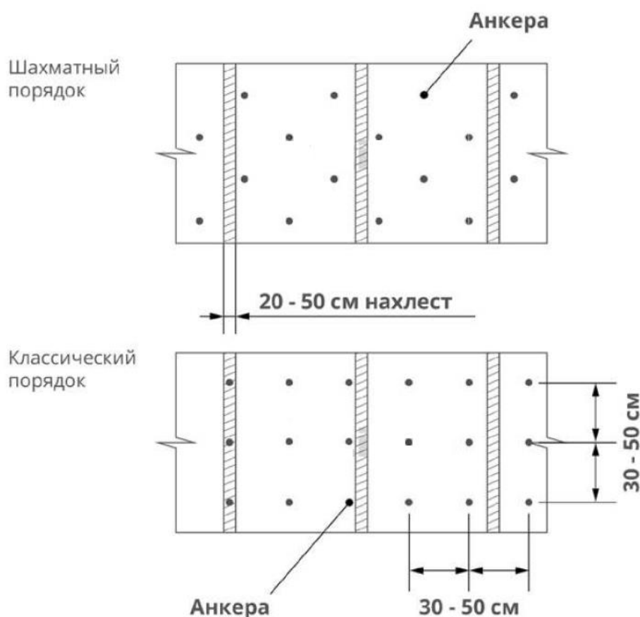
Рис. 5 – Схема анкеровки биоматов на поверхности склона
