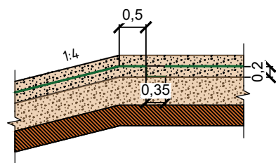
Узел Б. Анкерная траншея крепления биоматов
