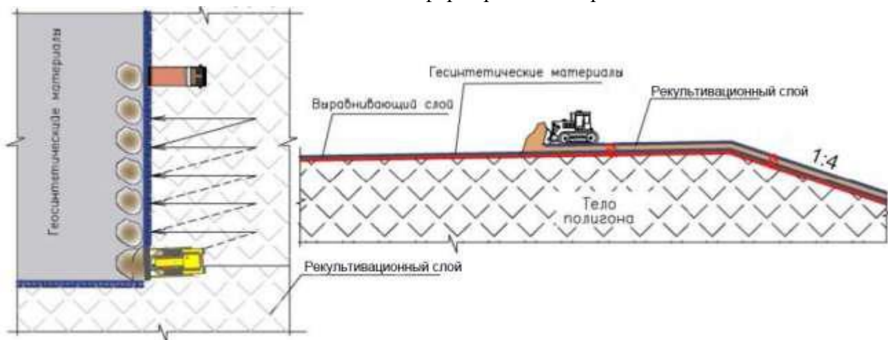
Рис. 3 – Условная схема формирования гидроизоляционного и защитного слоев
