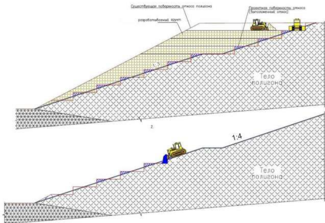
Рис. 1 – Условная схема выколаживания откосов
