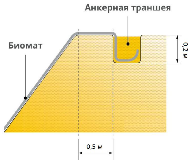
Рис. 6 – Схема анкерной траншеи
