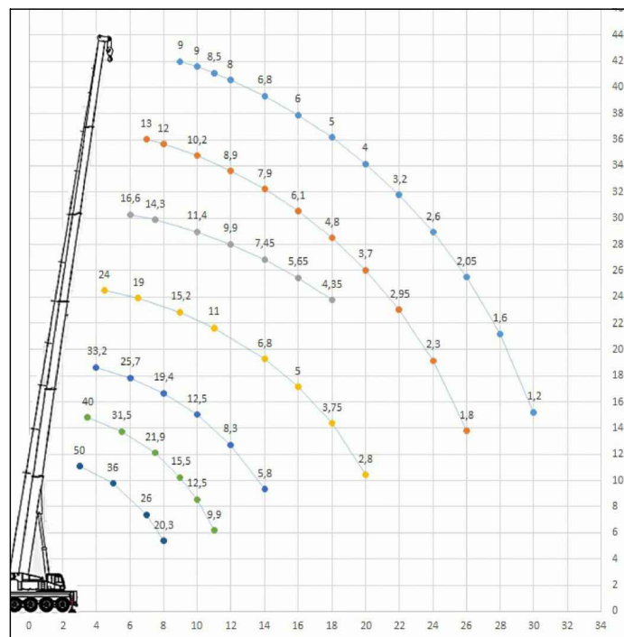
Грузовысотные характеристики крана XCMG XCT55_S
