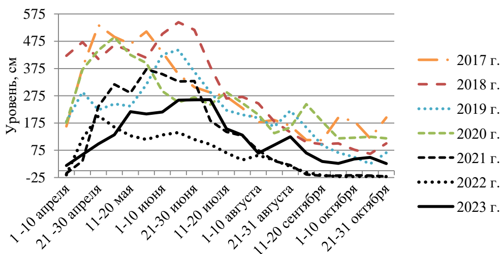
Рисунок 3 – Уровень воды в р. Обь в нижнем бьефе Новосибирской ГЭС
