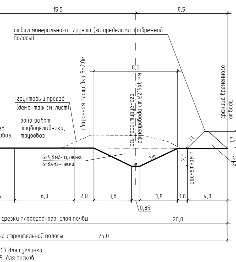
Тип 2 Полоса отвода на монтаж (линейная часть, береговая часть с расчетной глубиной 2,5 м)
