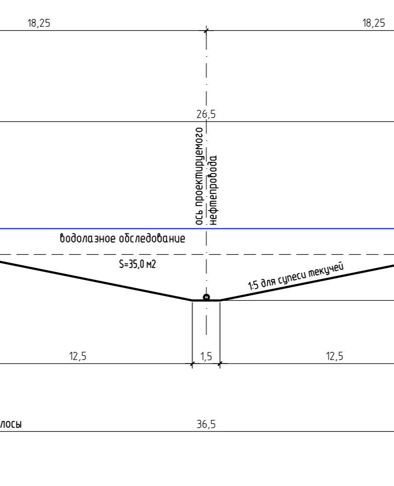
Тип 4 Полоса отвода на монтаж (подводная траншея с расчетной глубиной 2,5 м)
