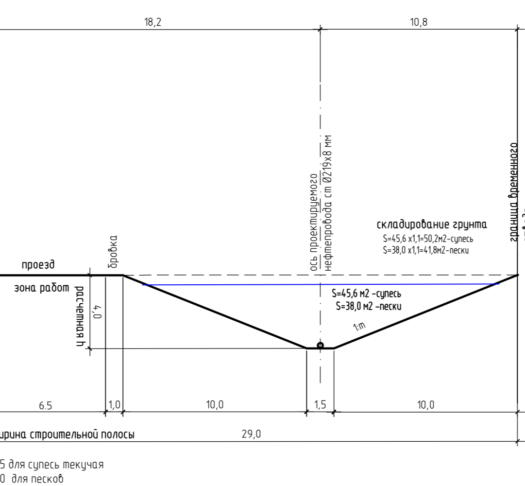
Тип 3 Полоса отвода на монтаж (береговая обводненная траншея с расчетной глубиной 4,0 м)
