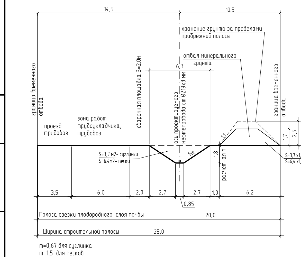
Тип 1 Полоса отвода на монтаж (линейная часть, береговая часть с расчетной глубиной 1,8 м)
