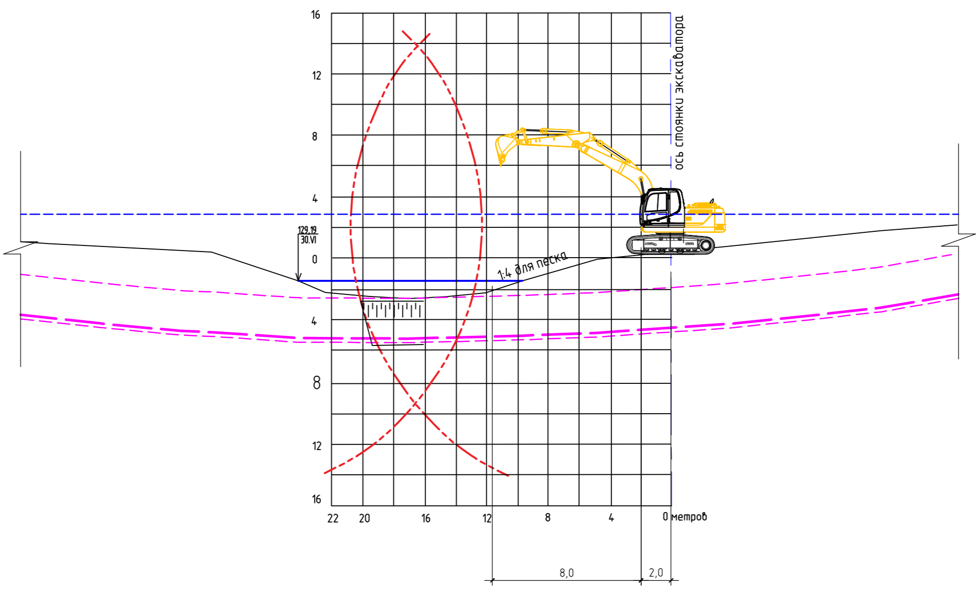
Схема разработки подводной траншеи экскаватором с удлиненной стрелой Hyundai R330LC-9S. Технические характеристики.
