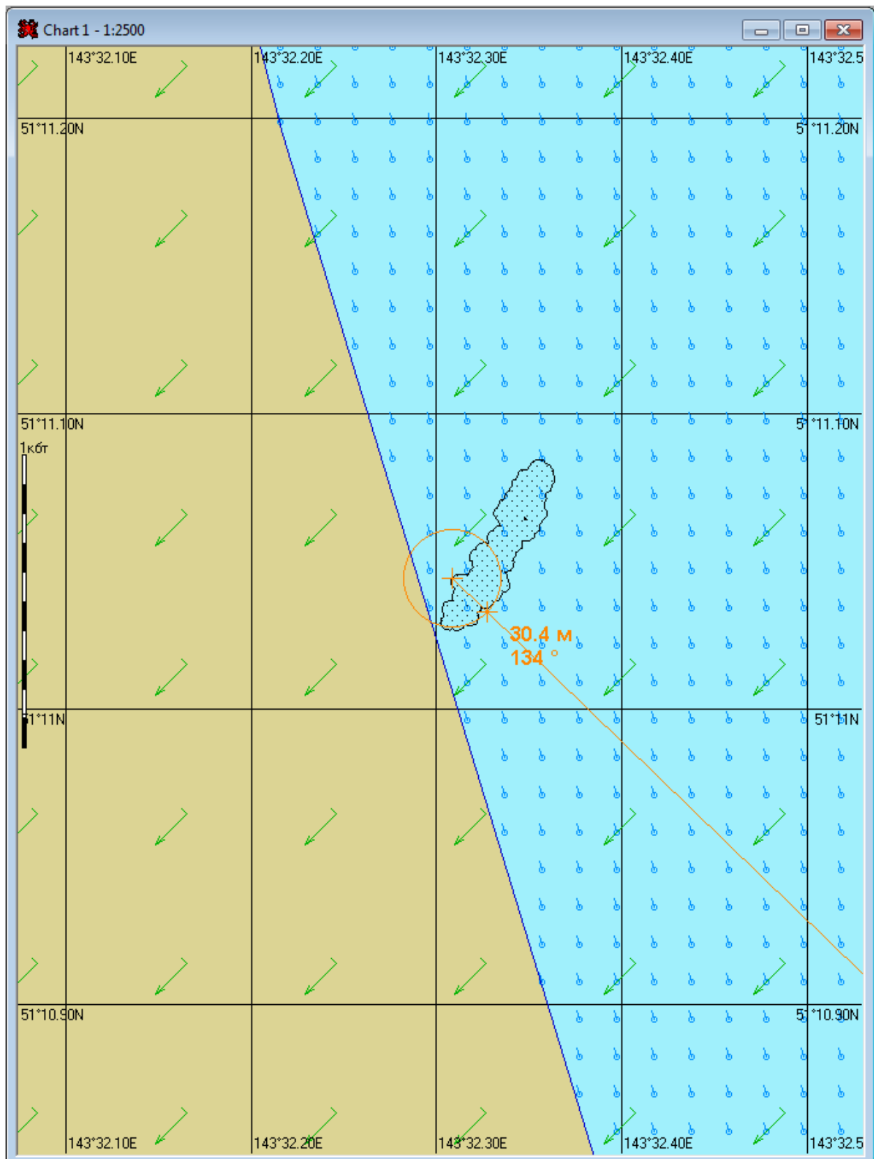
Рис. 2.7. Карта ЧС(Н) на момент достижения нефтяным пятном берега (29ч 05мин) при северо-восточном ветре и скорости ветра 5 м/с.
