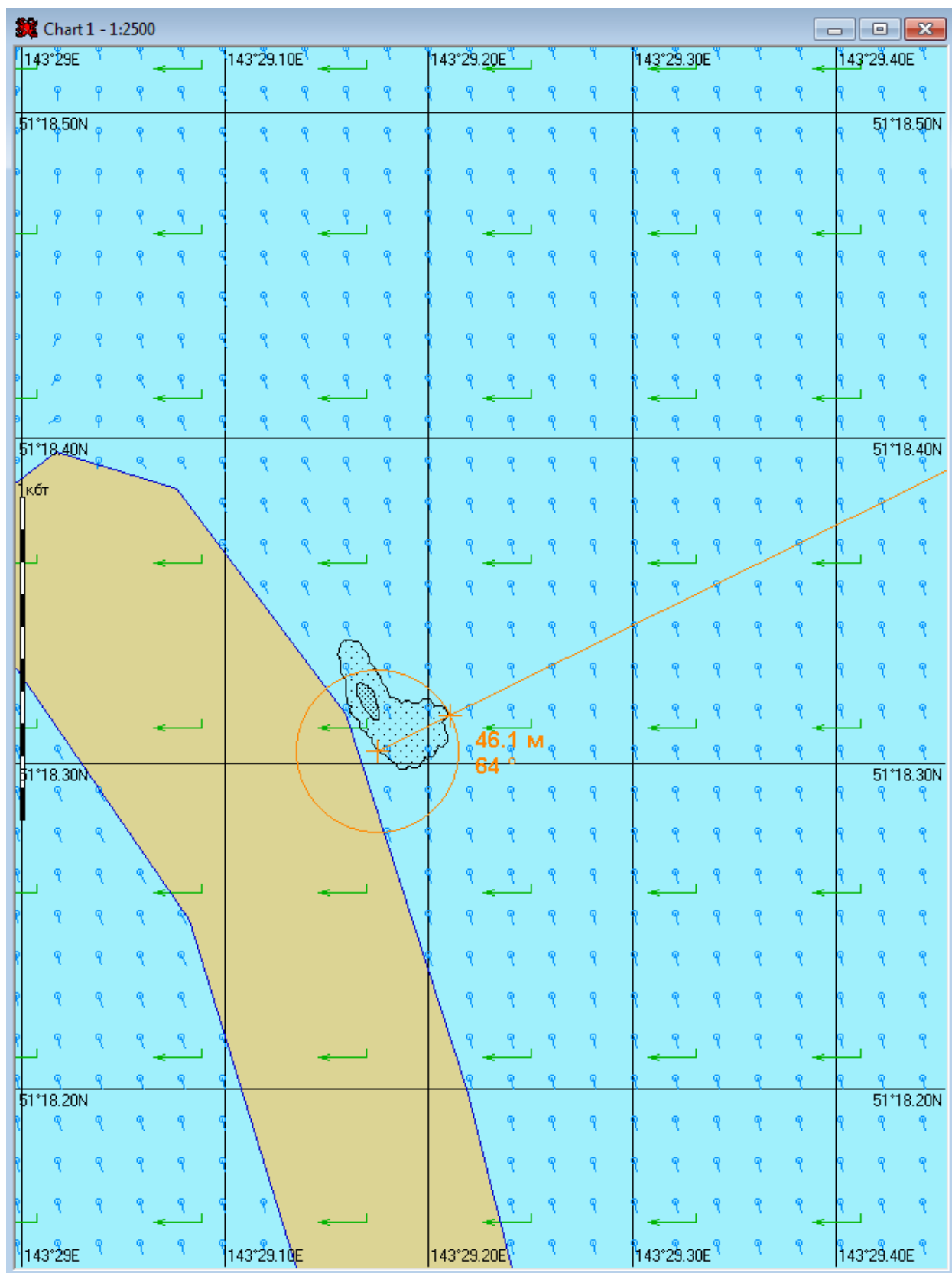
Рис. 2.6. Карта ЧС(Н) на момент достижения нефтяным пятном берега (24ч 50мин) при восточном ветре и скорости ветра 5 м/с.
