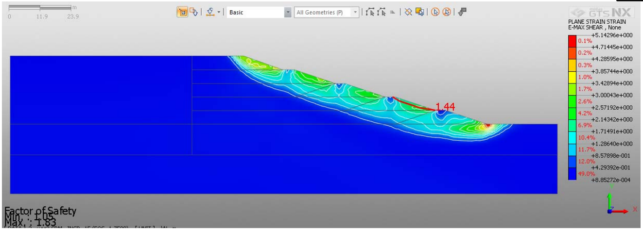
Рисунок 6.2 – Основной расчетный случай: Коэффициент устойчивости методом снижения прочности (SRM) -1,75, коэффициент устойчивости методом предельного равновесия (SAM) – 1,44
