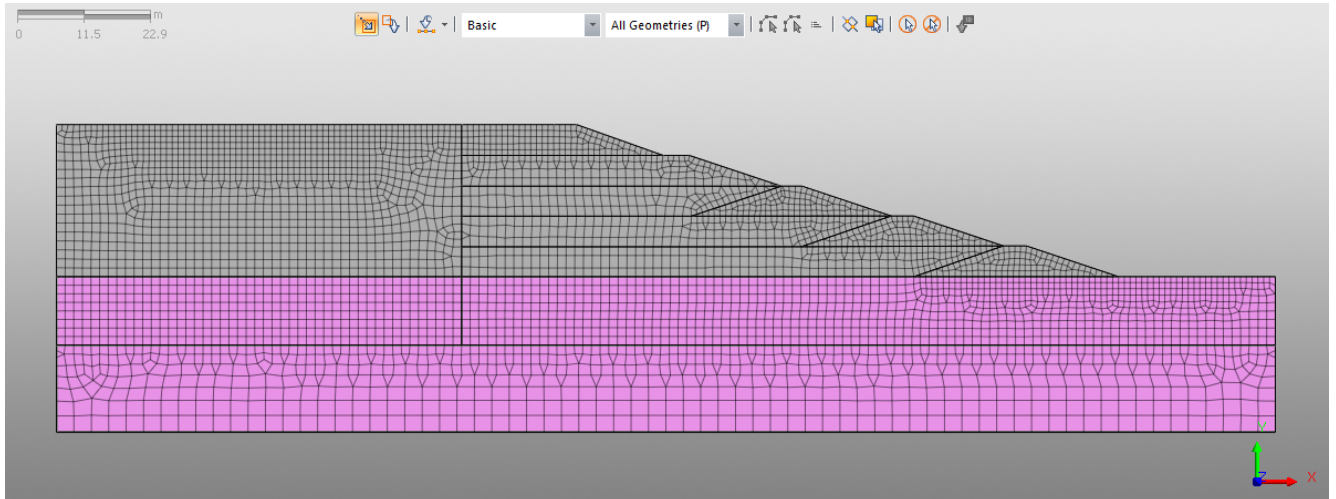
Рисунок 6.1 – Расчетная схема конечно-элементной модели
