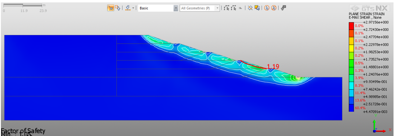
Рисунок 6.3 – Особый расчетный случай. Сейсмика 86: Коэффициент устойчивости методом снижения прочности (SRM) -1,475, коэффициент устойчивости методом предельного равновесия (SAM) – 1,19
