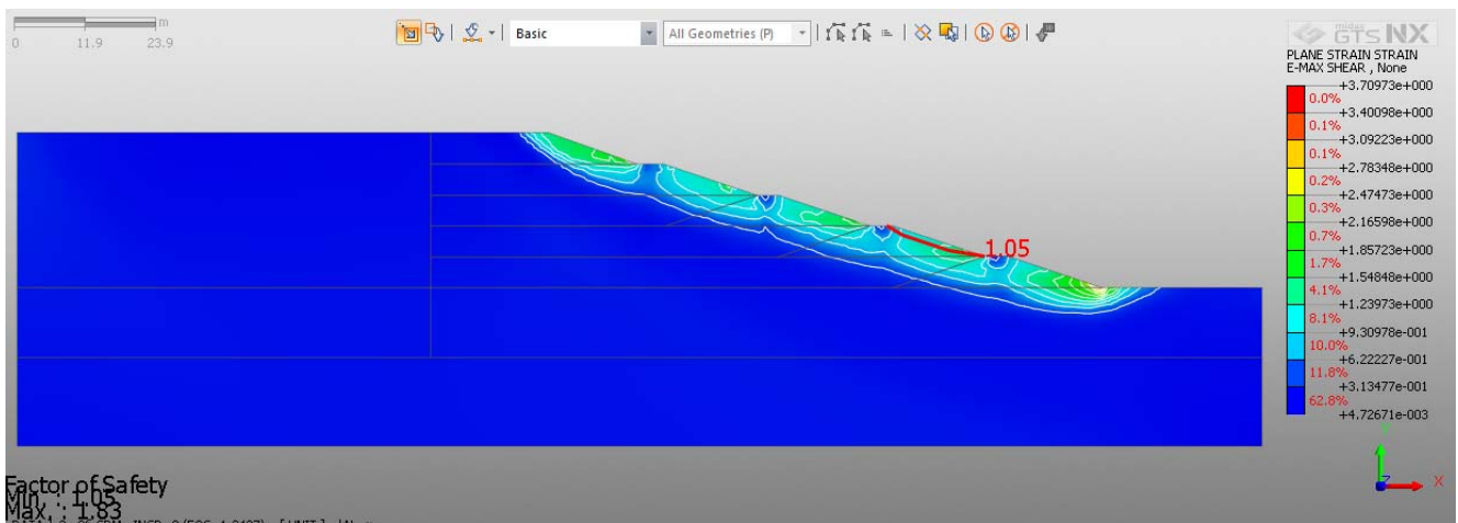
Рисунок 6.4 – Особый расчетный случай. Сейсмика 96: Коэффициент устойчивости методом снижения прочности (SRM) -1,243, коэффициент устойчивости методом предельного равновесия (SAM) – 1,05
