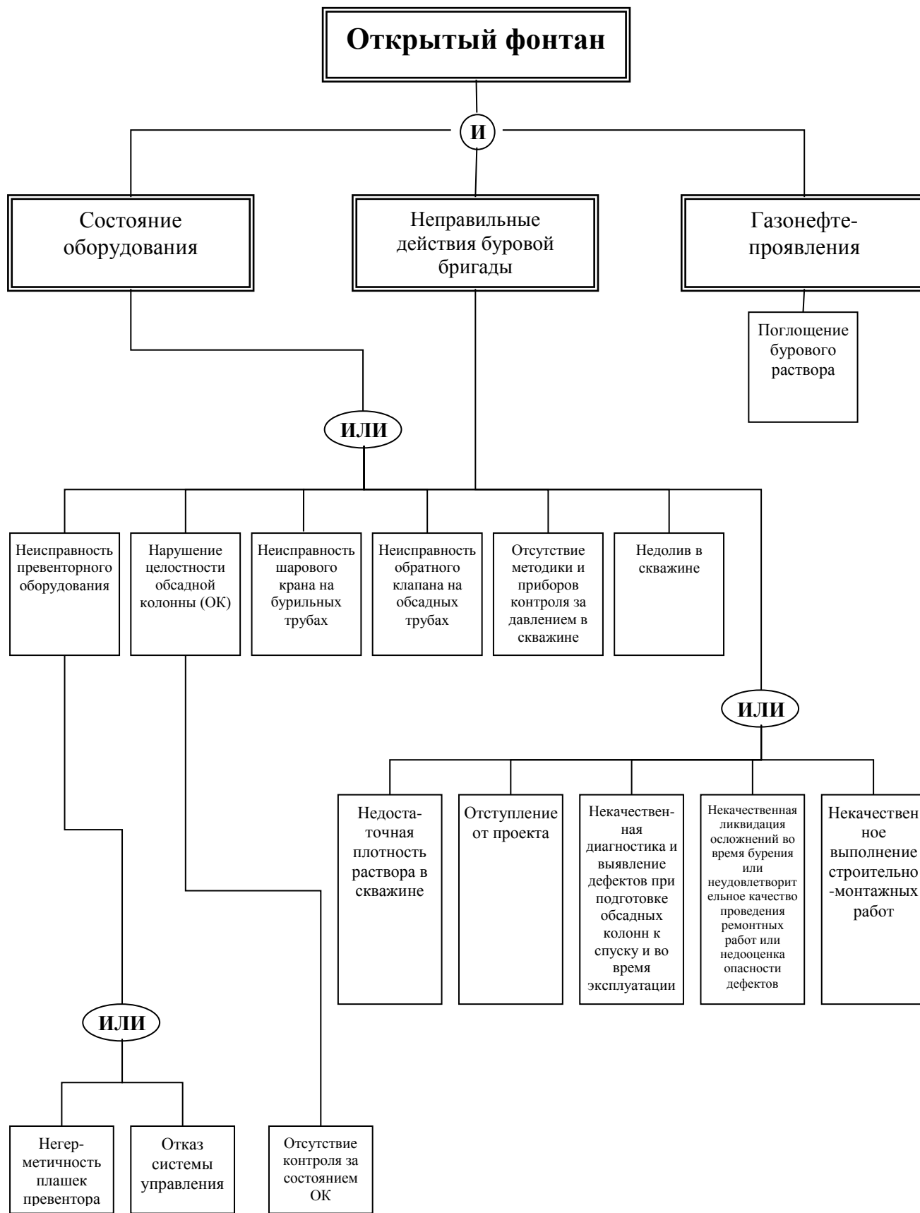
Рисунок 1 – «Дерево отказов»
