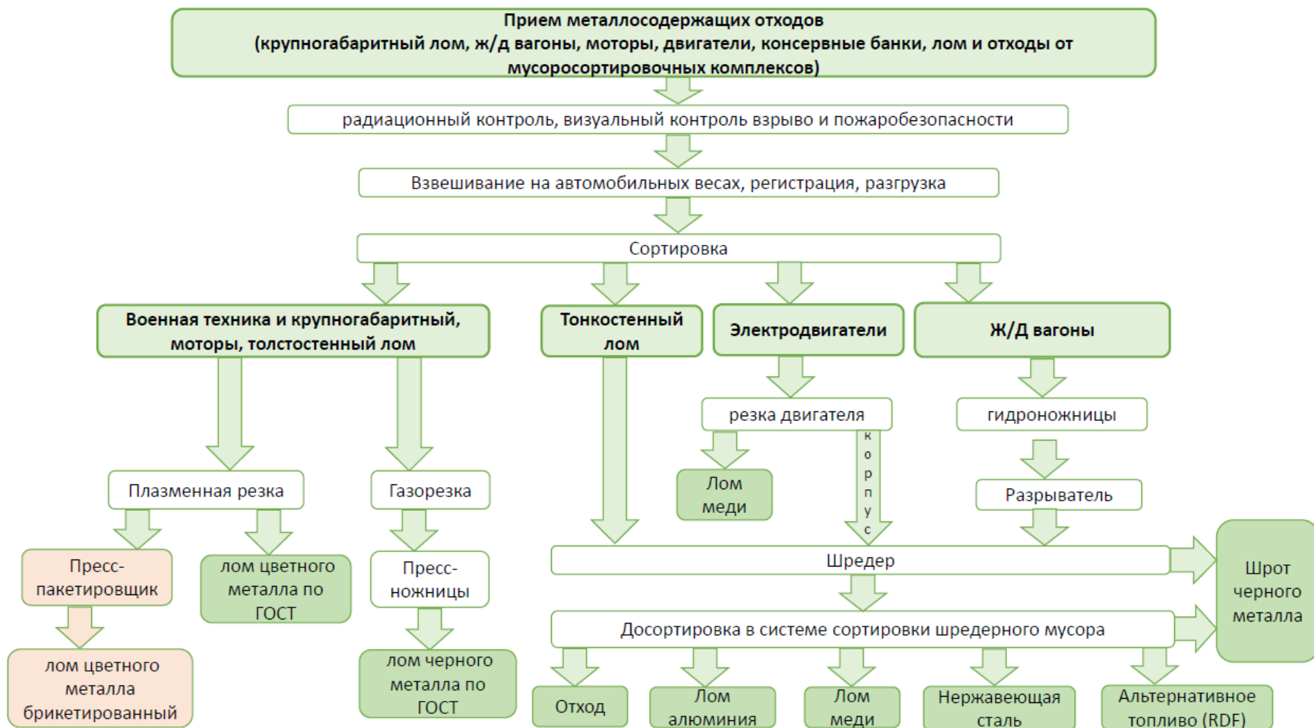
Рисунок 1.1 - Технологическая блок-схема
