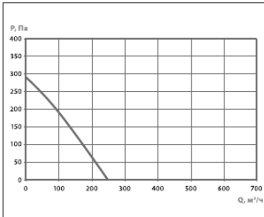
Канал-ВЕНТ-160
