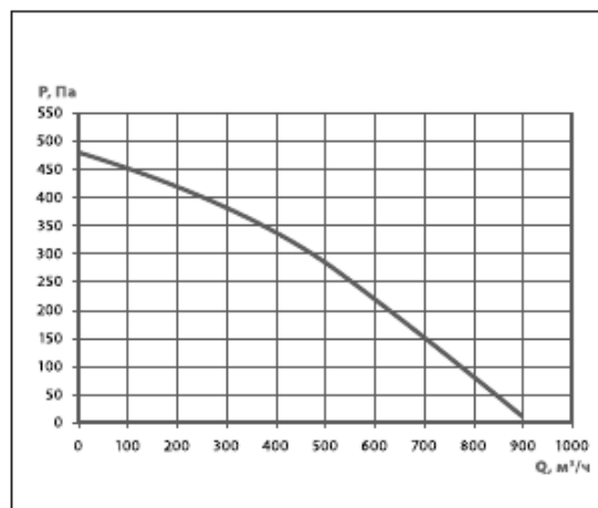
Канал-ВЕНТ-315
