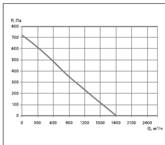
Канал-ВЕНТ-315
