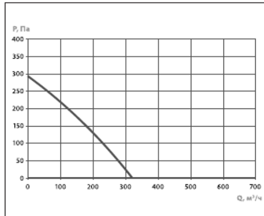
Канал-ВЕНТ-200
