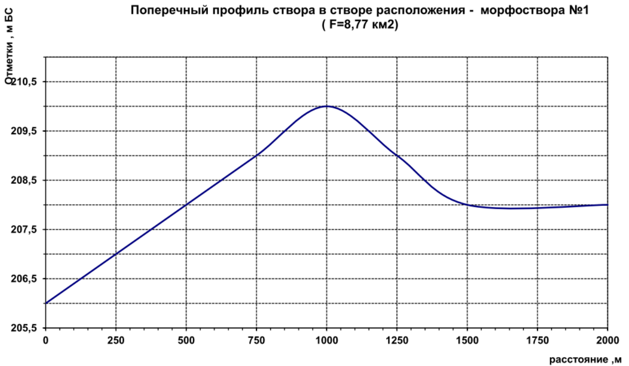
Рисунок 9.1 Поперечный профиль морфоствора
