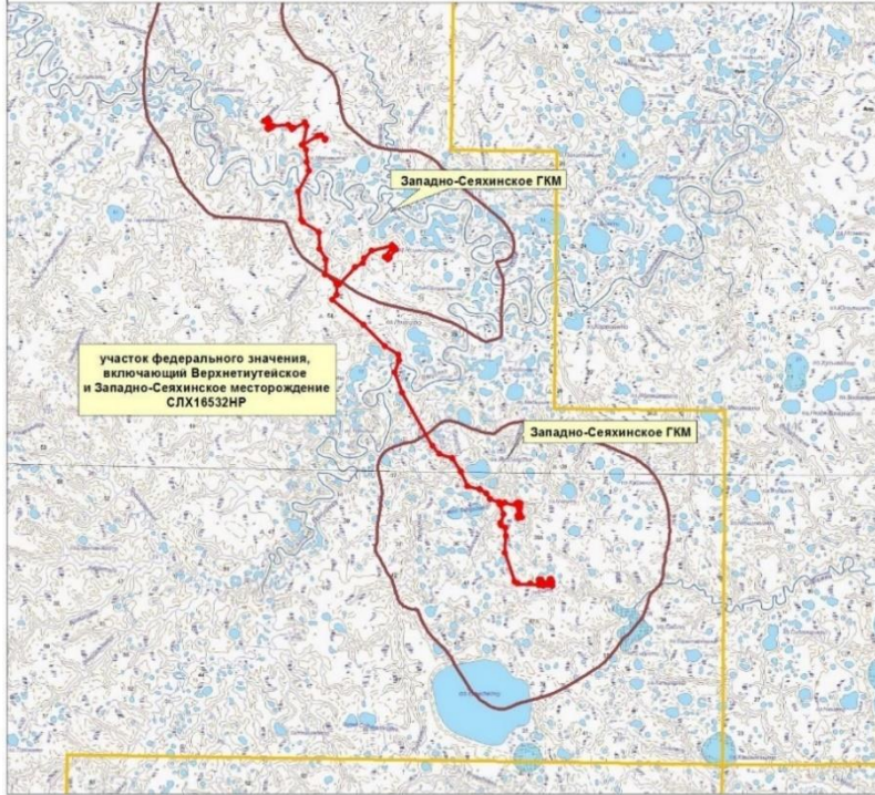
Схема расположения участка работ по объекту: "Обустройство Западно-Сеяхинского месторождения. Кусты скважин №№ 21, 22, 23, 11, 12, система газосбора" Масштаб 1:200 000
