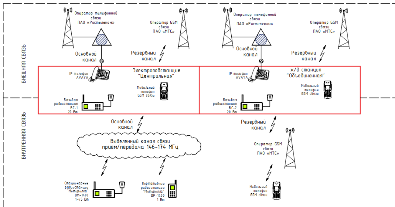
Рисунок 1.1 – Структурная схема системы связи
