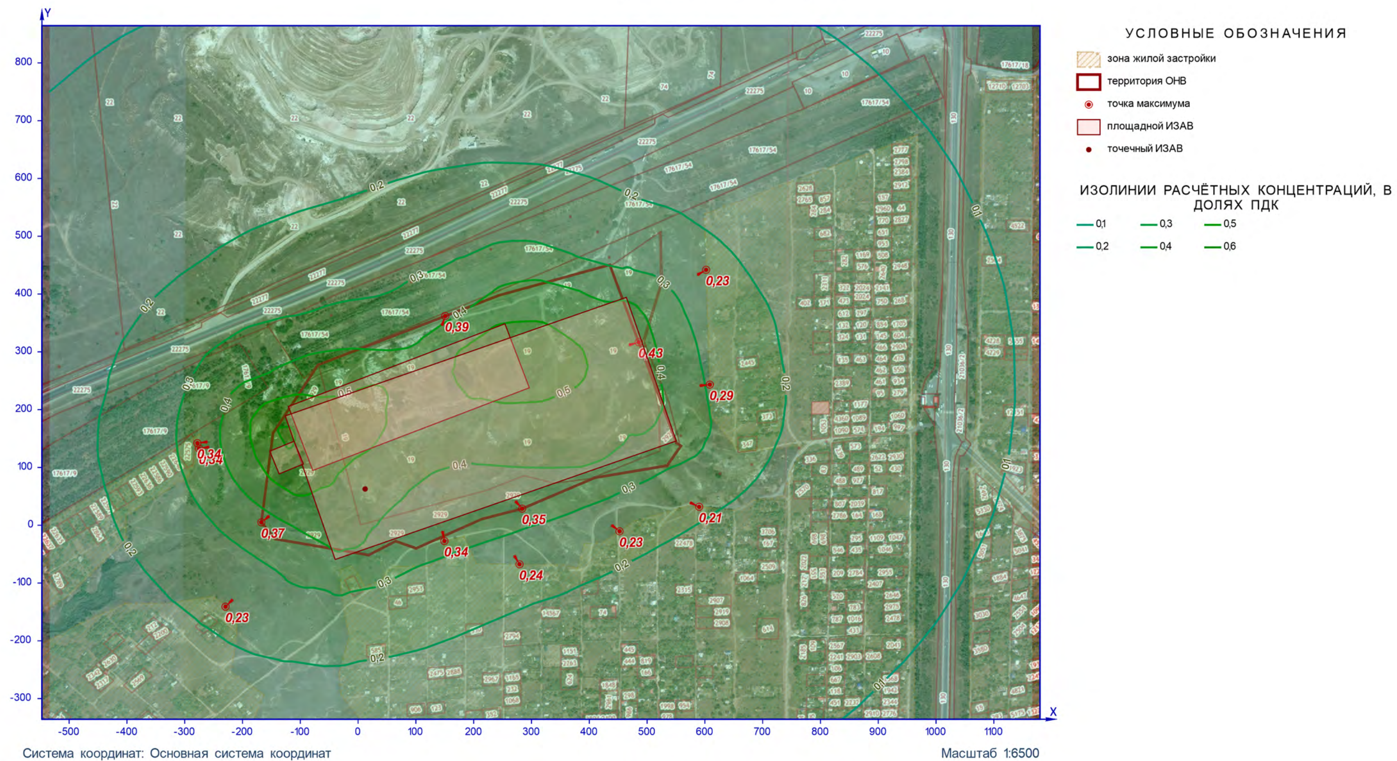
Рисунок 24 – Ситуационный план
