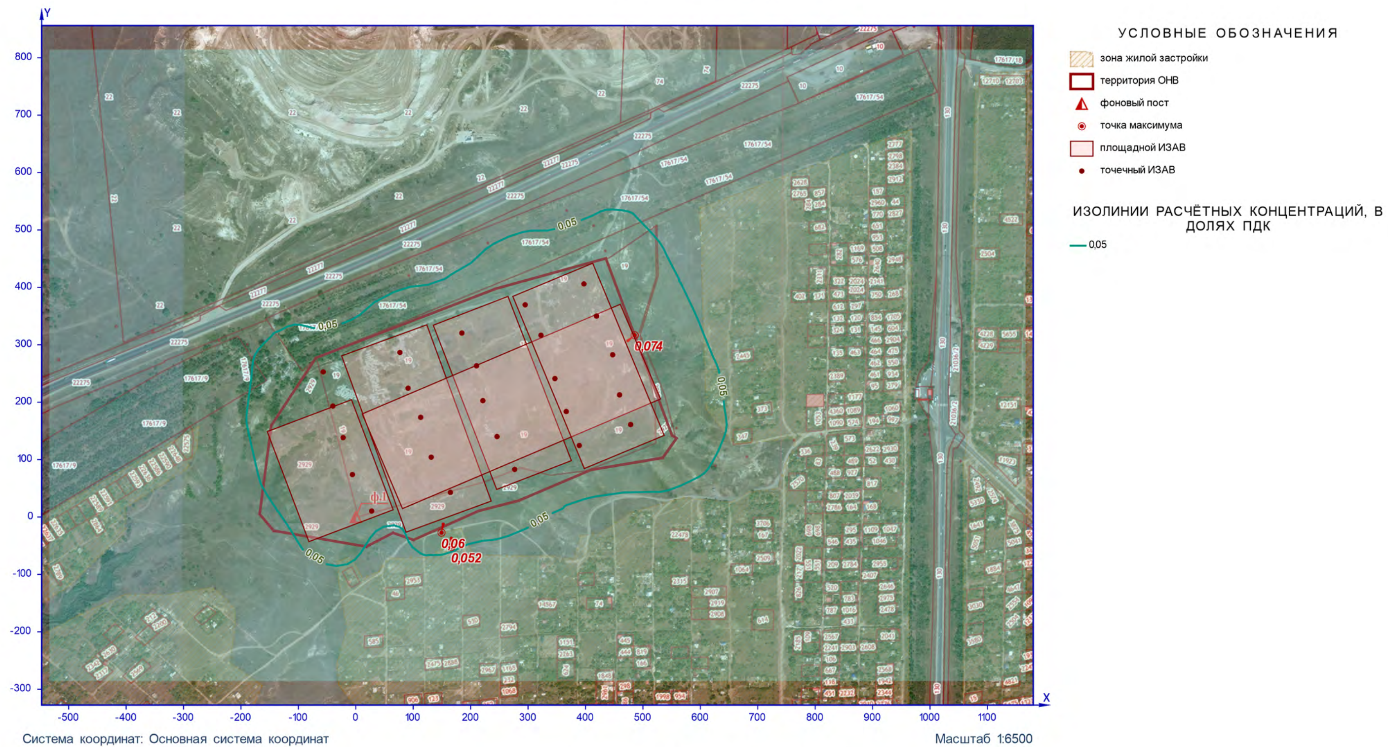
Рисунок 18 – Ситуационный план
