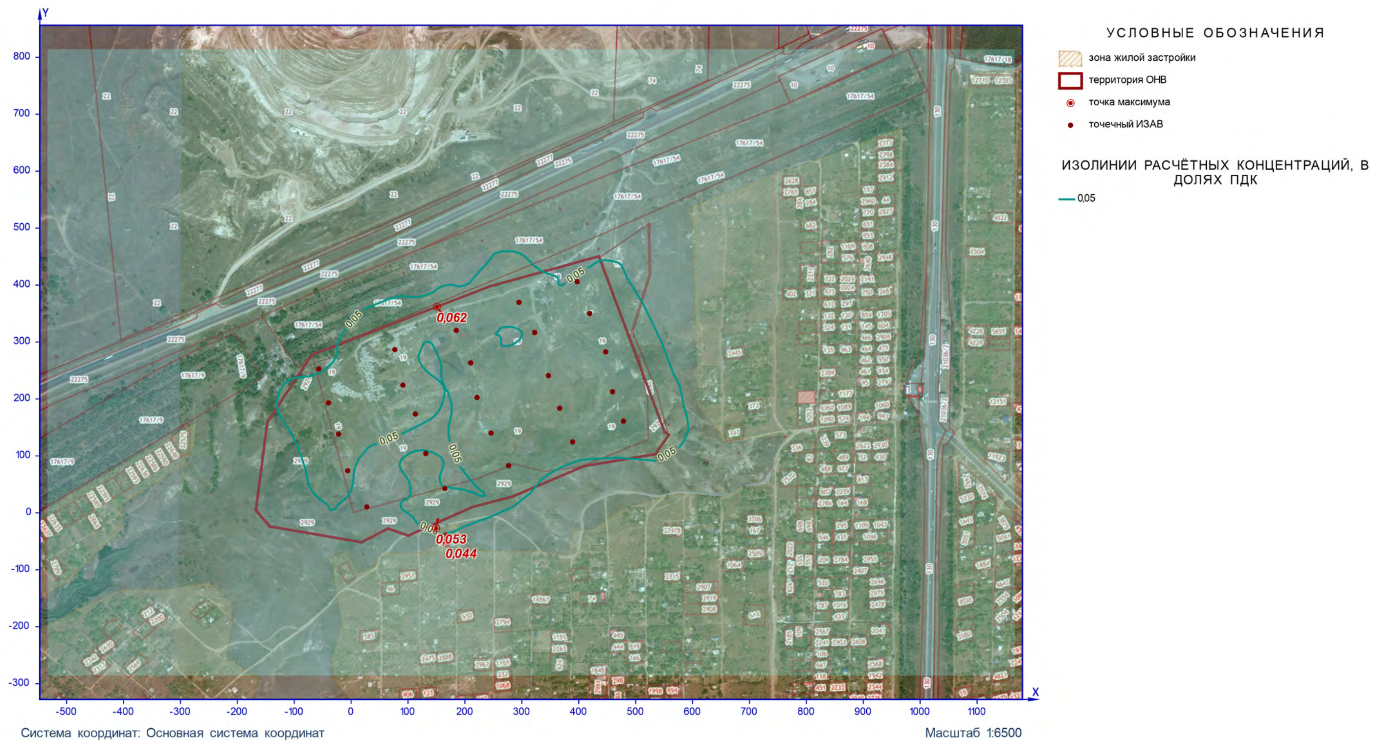
Рисунок 6 – Ситуационный план
