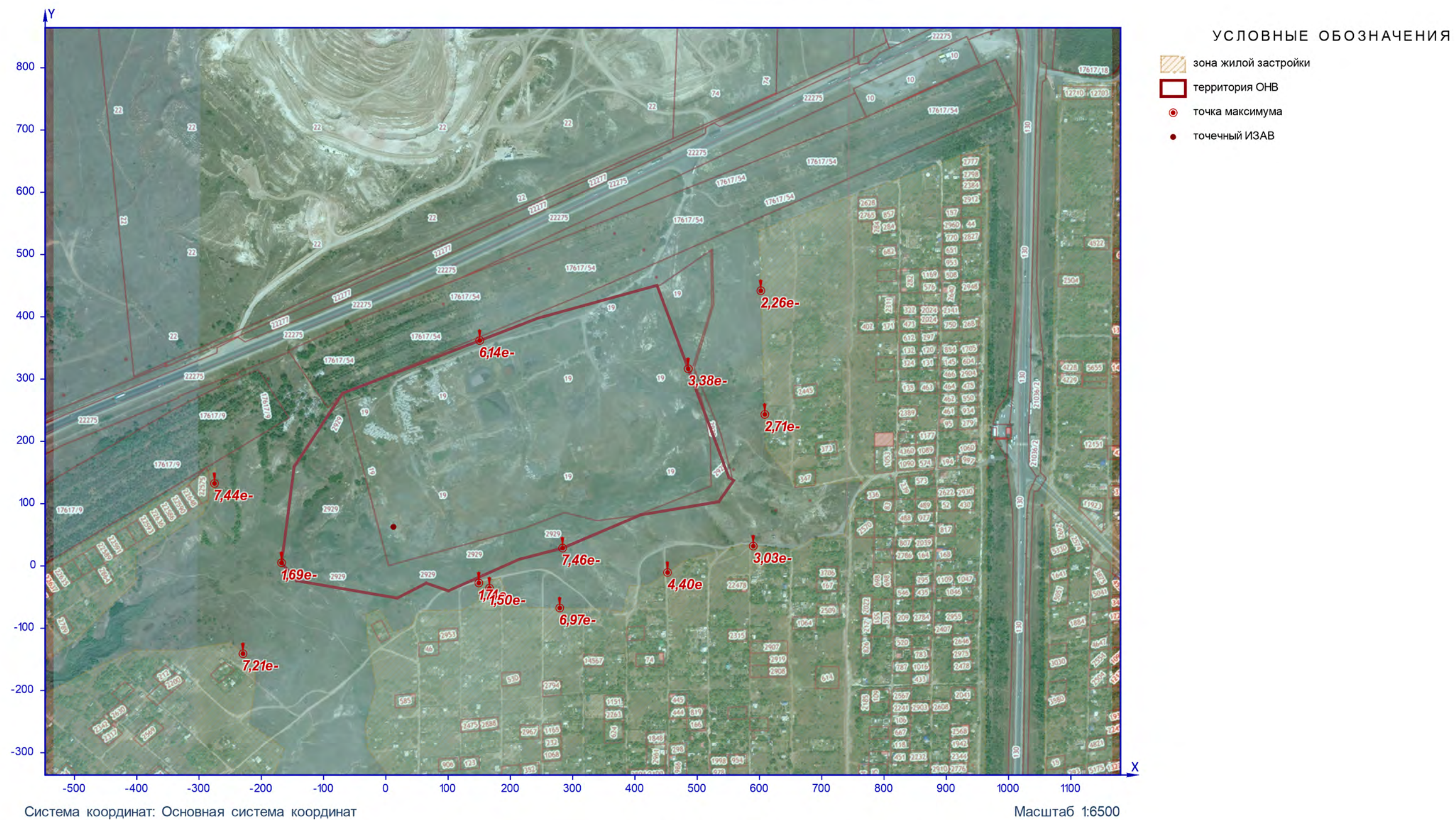
Рисунок 13 – Ситуационный план
