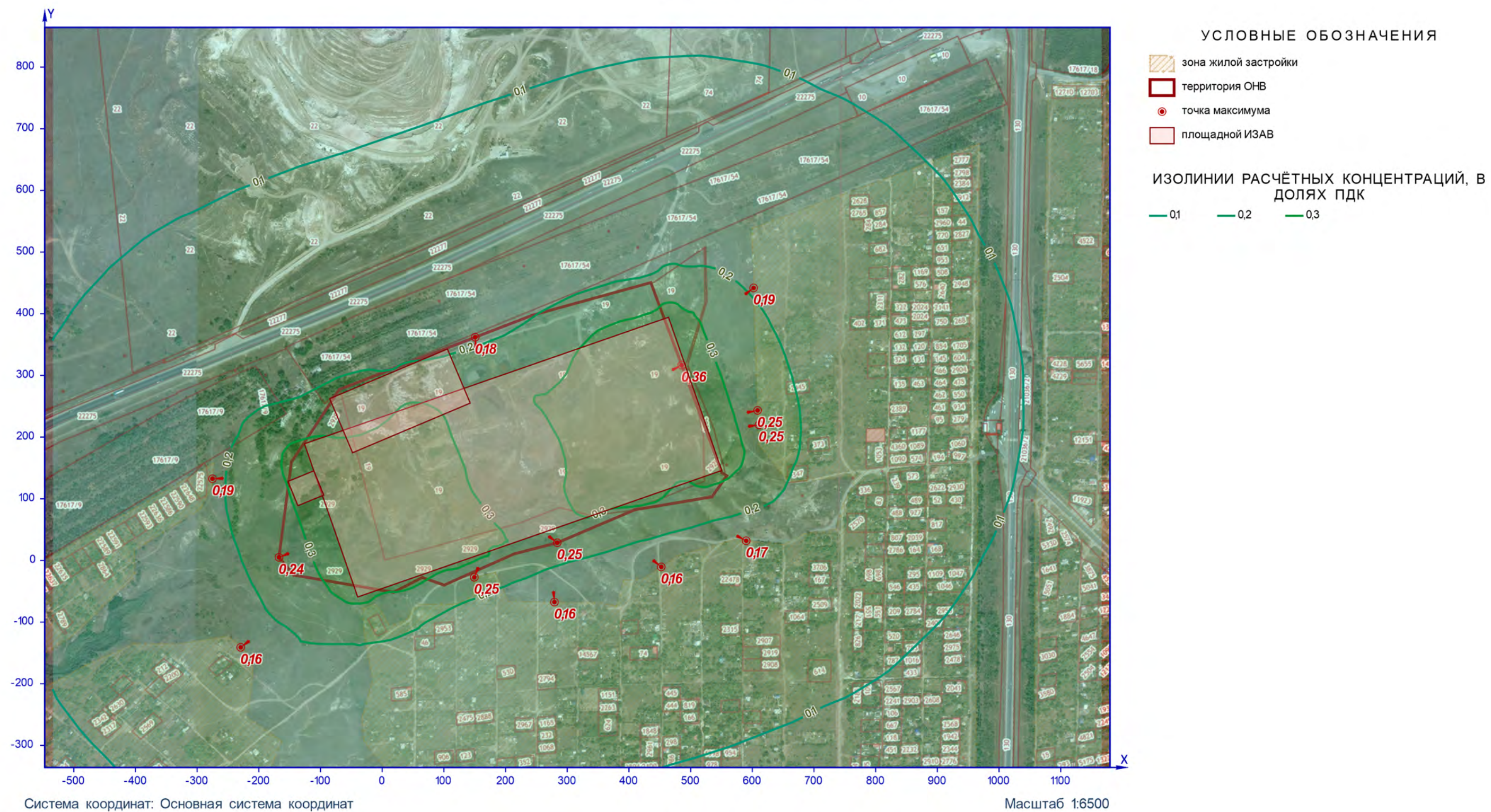
Рисунок 22 – Ситуационный план
