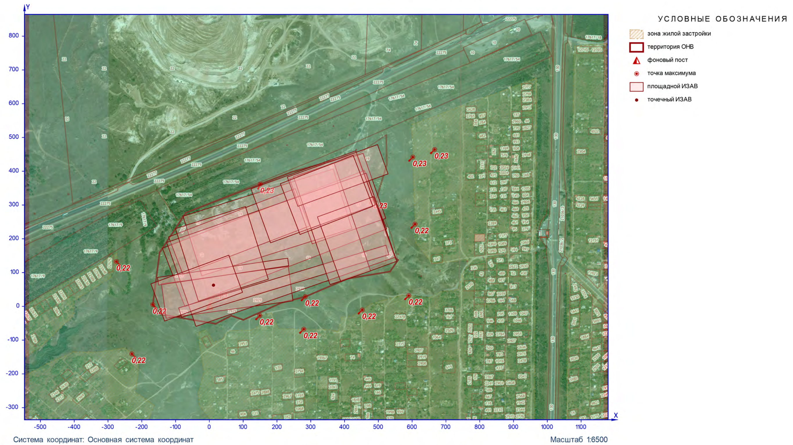
Рисунок 7 – Ситуационный план
