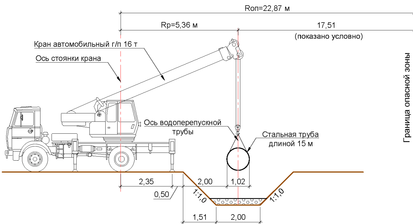
Рисунок Б.4 – Граница опасной зоны работы крана при монтаже стальной водоперепускной трубы
