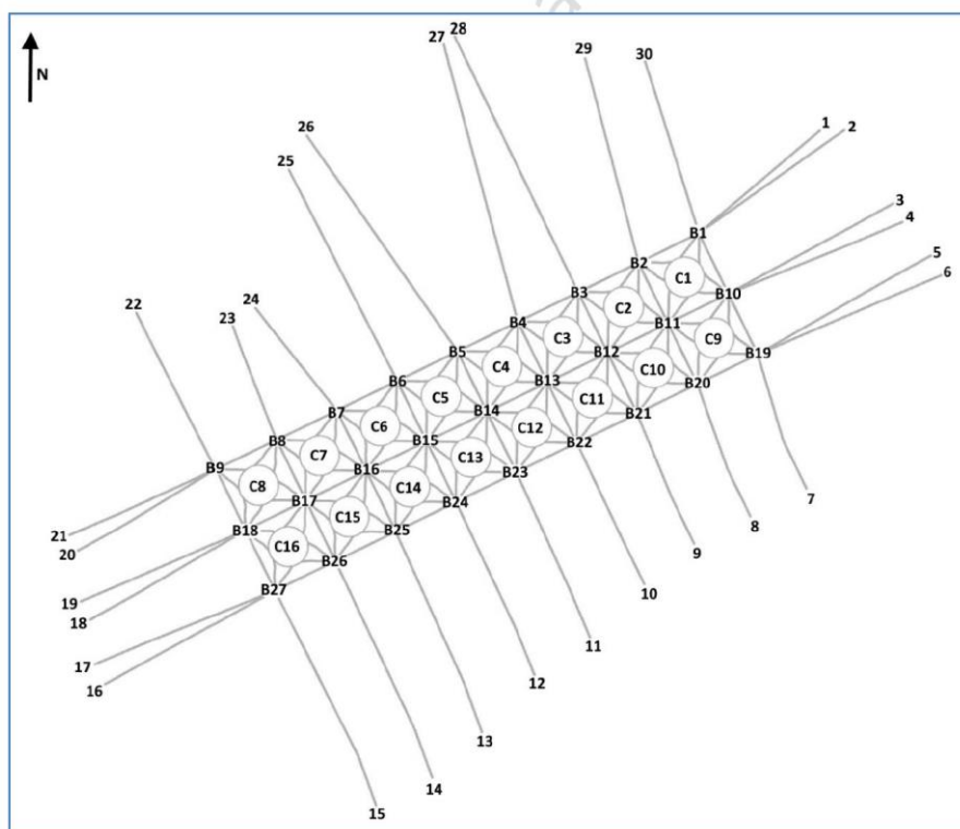
Рисунок 2.3 - Якорная система садкового комплекса
