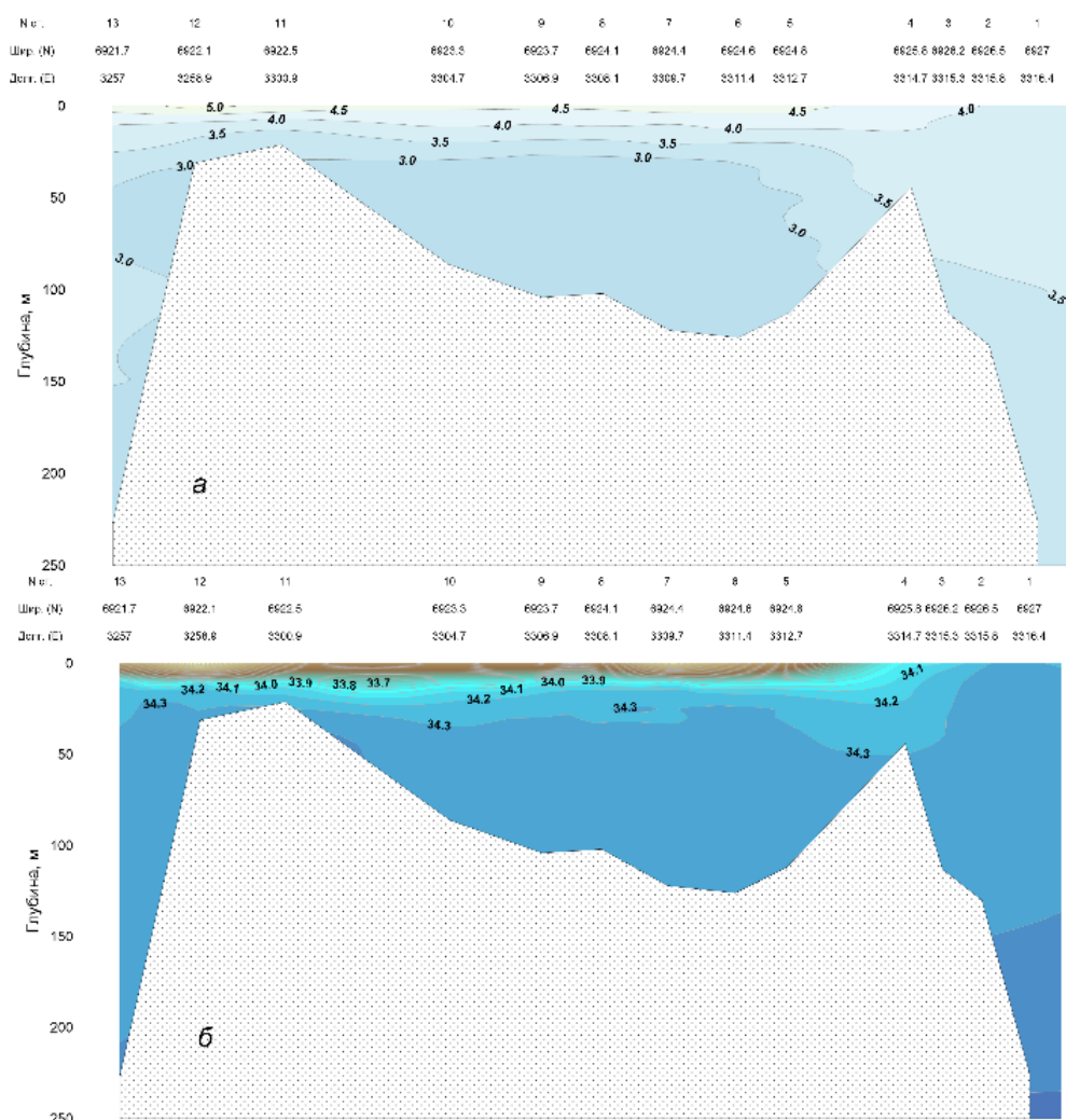
Рисунок 6.5 – Вертикальное распределение температуры (а) и солёности (б) вод на акватории Восточного рукава губы Ура весной (на примере наблюдений в мае 2017 г.)
