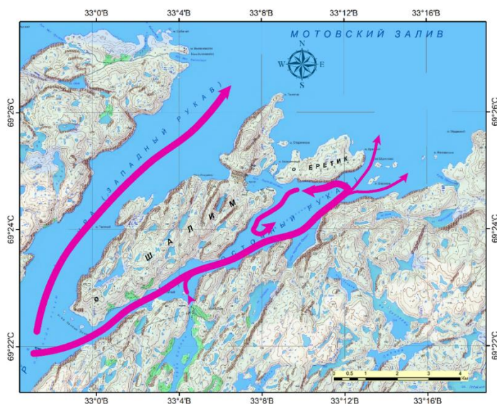
Рисунок 6.8 – Схематическая циркуляция вод в северной части губы Ура
