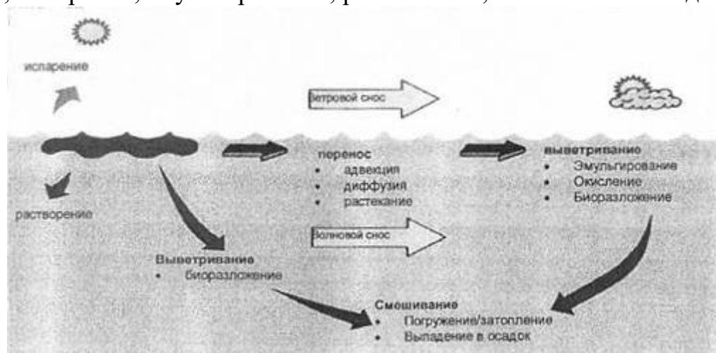
Рисунок 10.1 – Поведение дизельного топлива на воде
