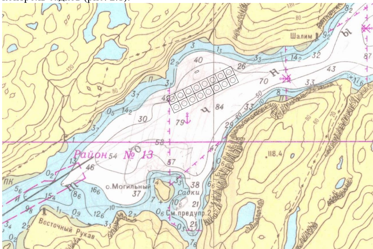
Рисунок 2.1 - Расположение СК и баржи в границах рыбоводного участка «Восточный рукав губы Ура («Шалим»)»
