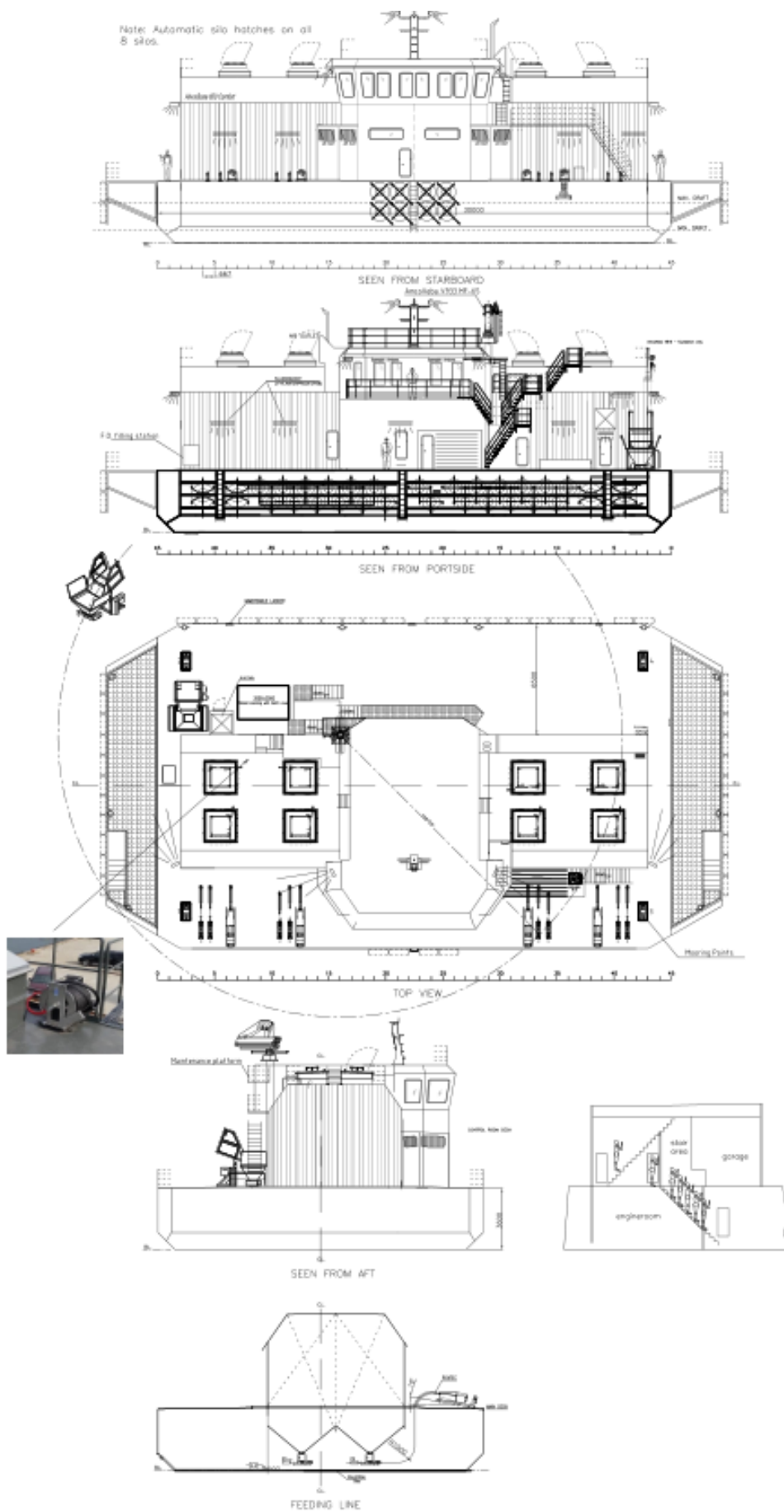
Рисунок 2.6 – Схема баржи Aqua BASE 650 Comfort
