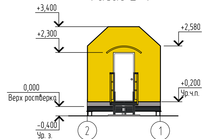
Фасад 2-1
