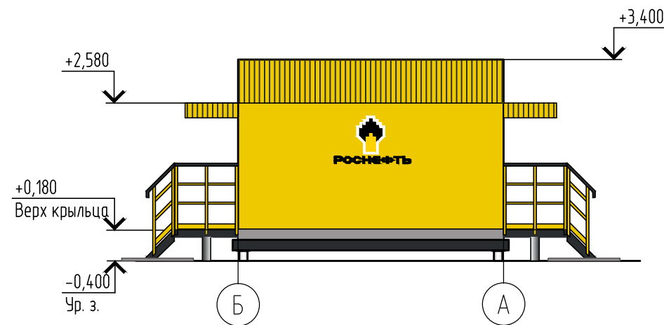
Фасад Б-А
