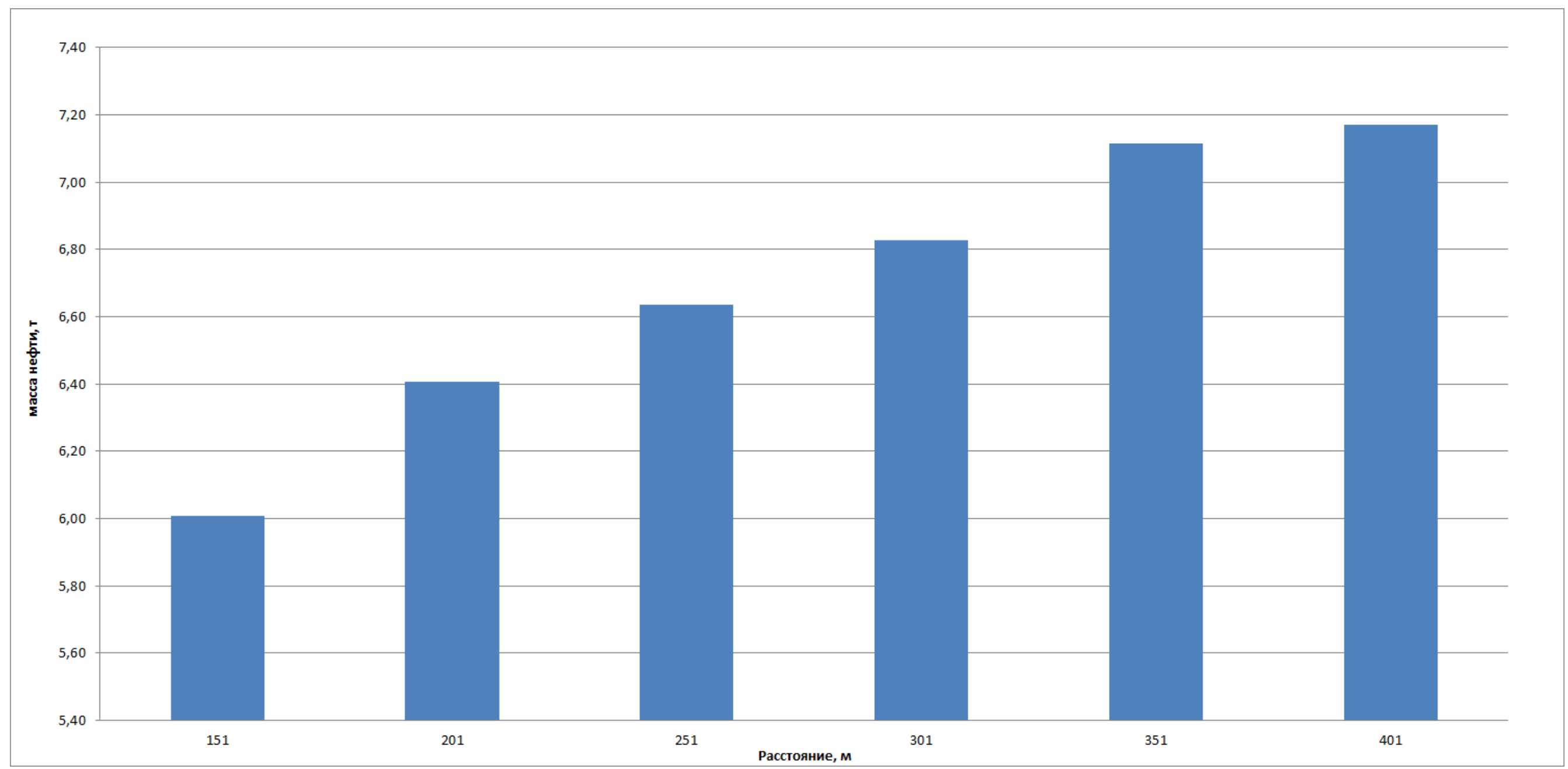
Рисунок 7 – Результаты расчетов количества опасных веществ, участвующих в аварии на нефтегазосборном трубопроводе, при возникновении свища
