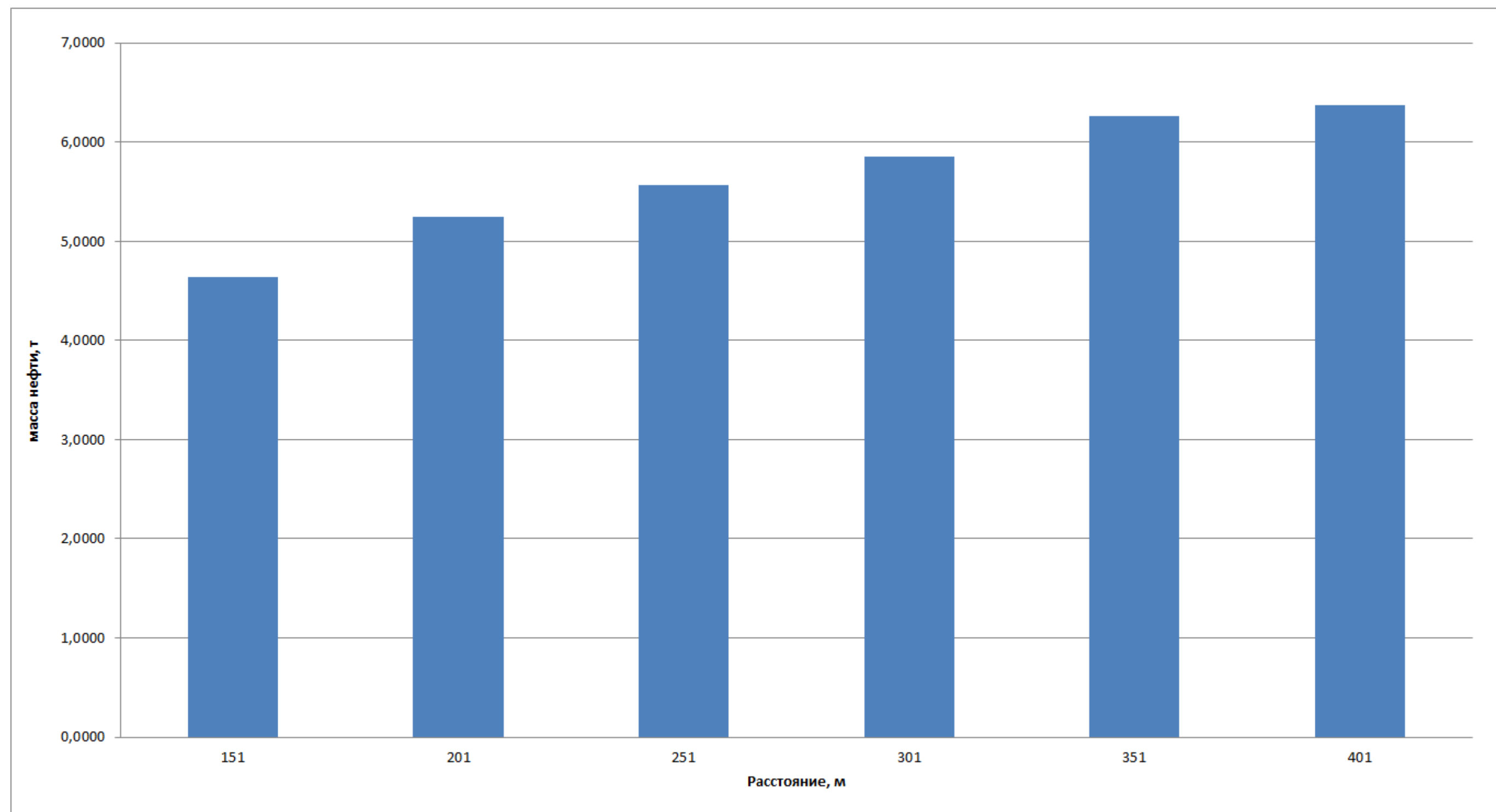
Рисунок 6 – Результаты расчетов количества опасных веществ, участвующих в аварии на нефтегазосборном трубопроводе, при гильотинном разрыве
