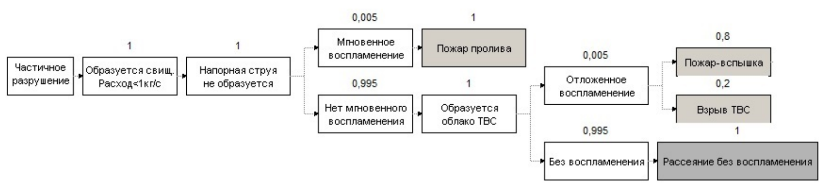
Рисунок 15 – Дерево событий при частичном разрушении на нефтесборных трубопроводах (горючая жидкость и газ)
