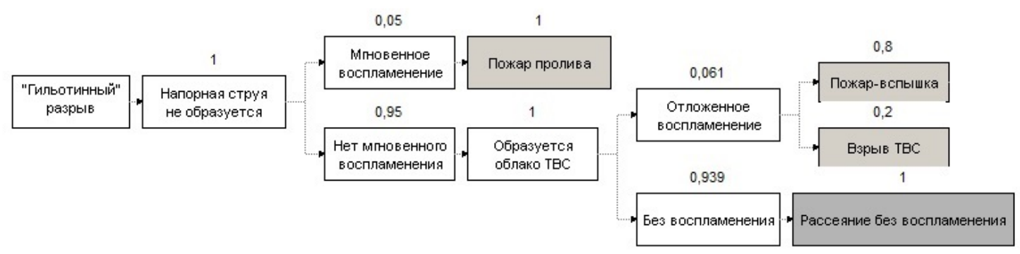
Рисунок 14 – Дерево событий при полном разрушении на нефтесборных трубопроводах (горючая жидкость и газ)
