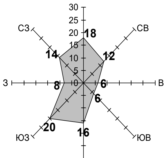
Рисунок 2.2 - Среднегодовая роза ветров за теплый период года (апрель-октябрь) на метеостанции «Зашеек»
