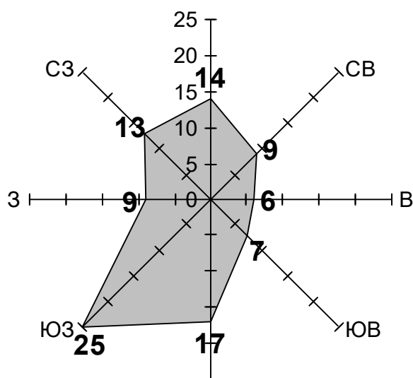
Рисунок 2.3 - Среднегодовая роза ветров на метеостанции «Зашеек»
