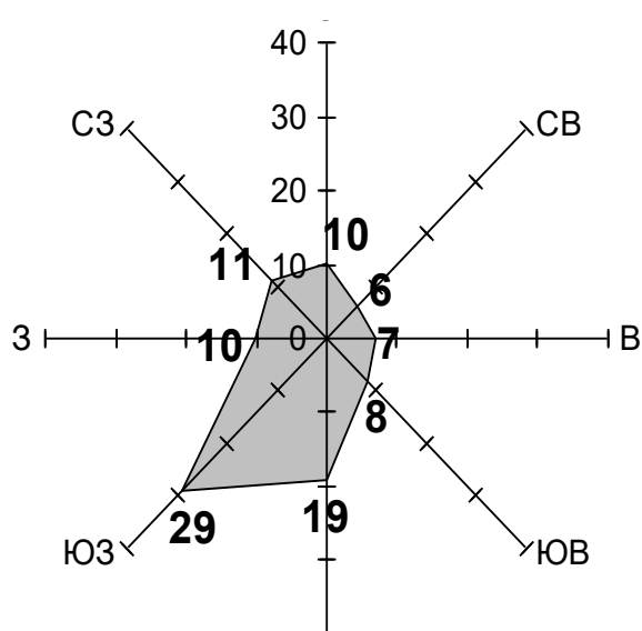
Рисунок 2.1 - Среднегодовалая роза ветров за холодный период года (ноябрь-март) на метеостанции «Зашеек»
