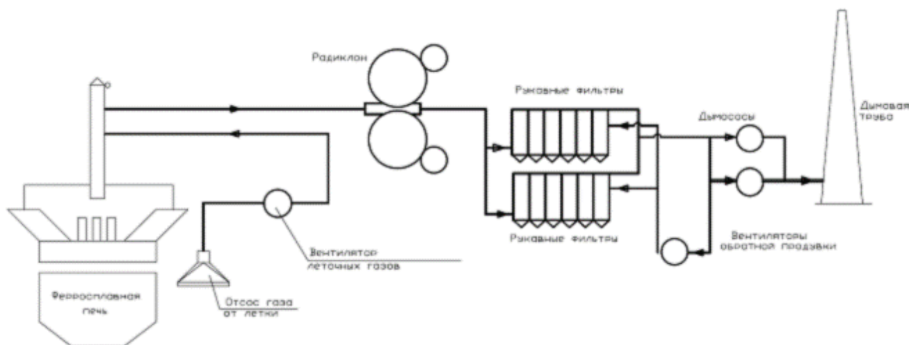
Рисунок 2.3.1-1. Технологическая схема газоочистки печей №№ 11, 12, 13, 15 (для одной печи)
