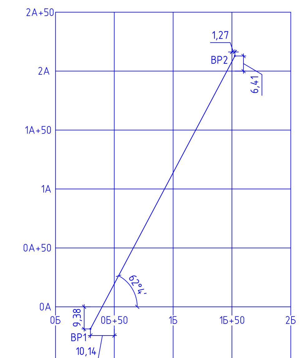
Схема привязки строительной сетки
